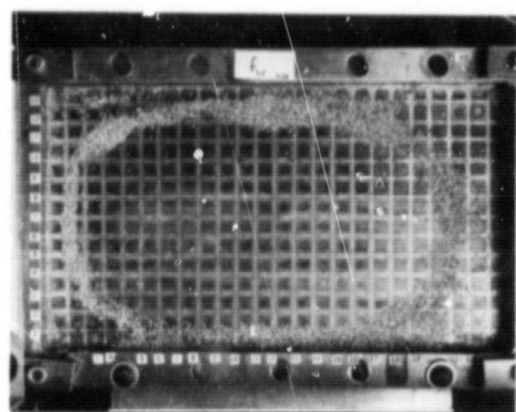
Mode (1,1)
