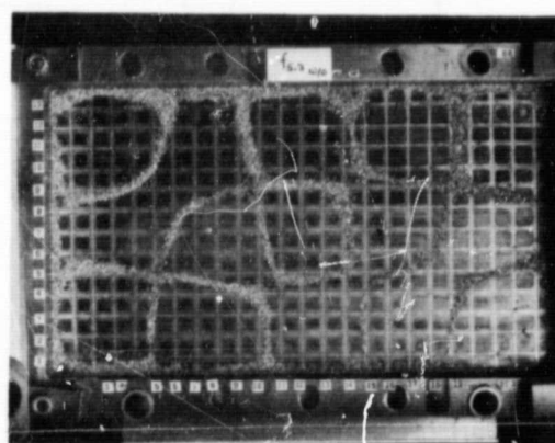
Mode (5,3)
