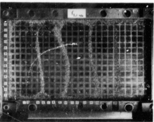
Mode (5,1)
