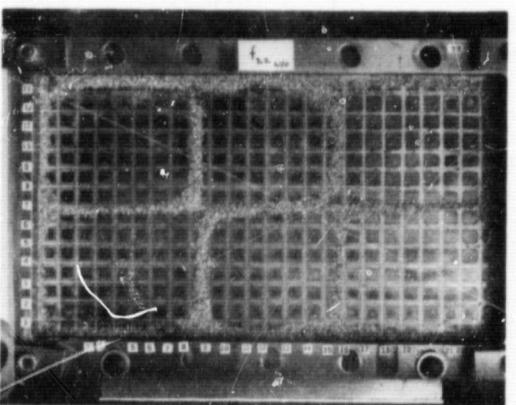
Mode (3,2)
