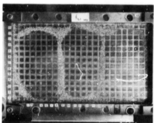
Mode (3,1)
