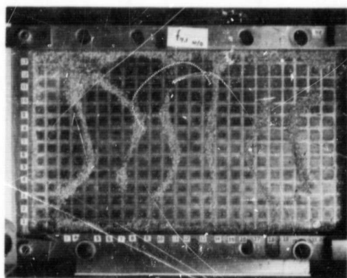
Mode (7,1)
