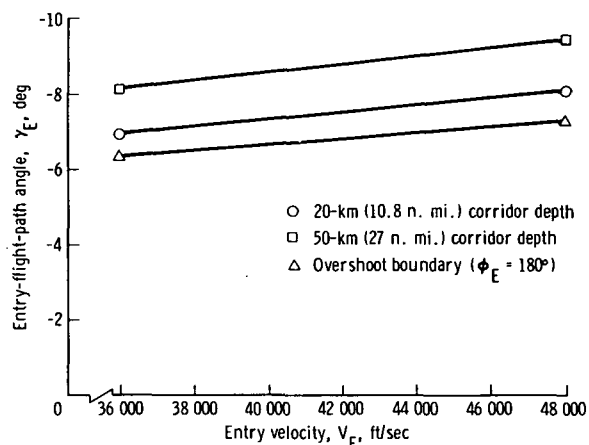
(d) L/D = 0.25 , M/C_D A = 1.0 \text{ slug/ft}^2 .
