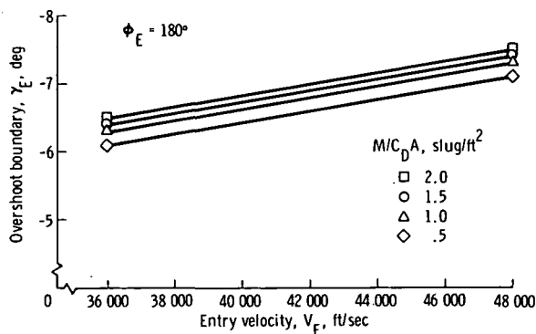
(b) L/D = 0.25 .
