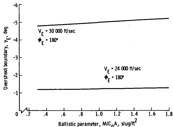
(b) L/D = 0.25 .
