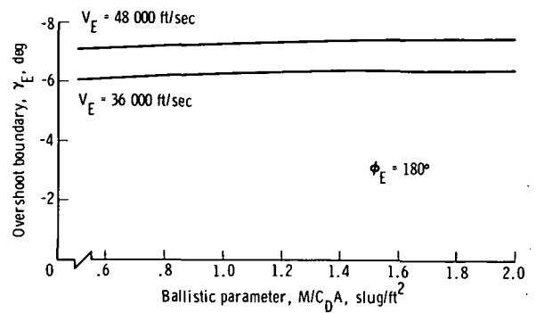
(b) L/D = 0.25 .
