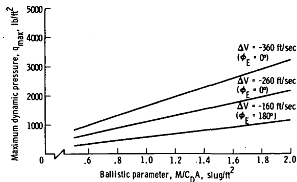
(b) L/D = 0.25 .
