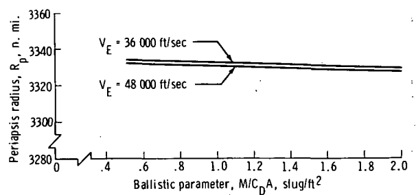
(b) L/D = 0.25 .
