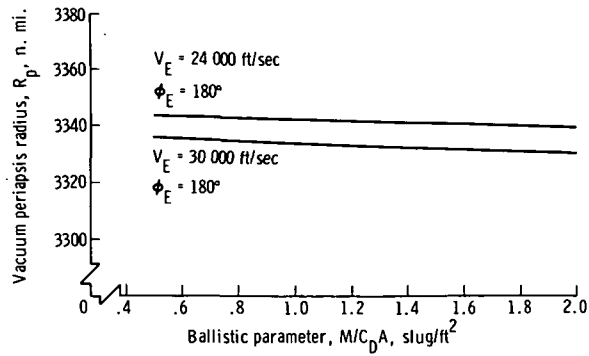
(b) L/D = 0.25 .
