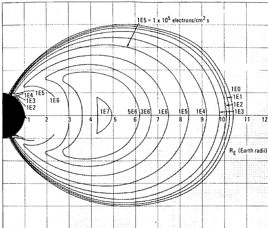
a. E > 0.5 MeV
