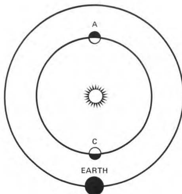
INFERIOR PLANETS
