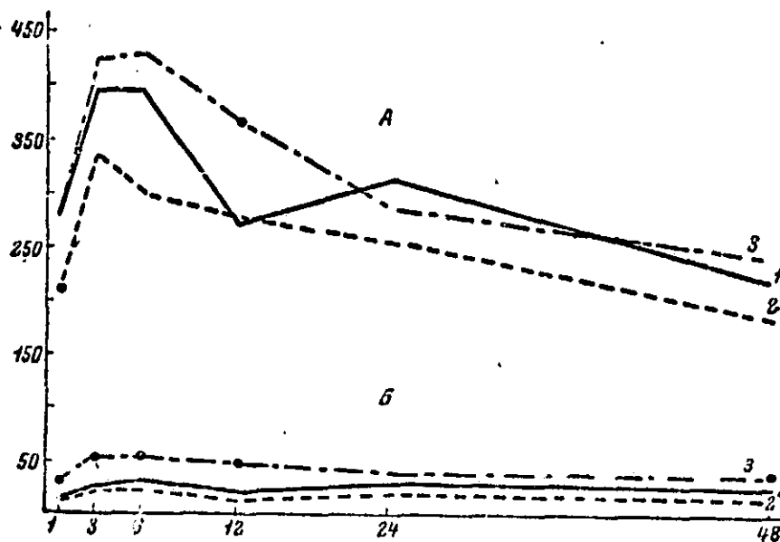
Рис. 2. Интенсивность включения радиоаминокислот- ^{14}\text{C} в белки тканей почек (А) и скелетных мышц (Б) крыс при различных режимах двигательной активности.
