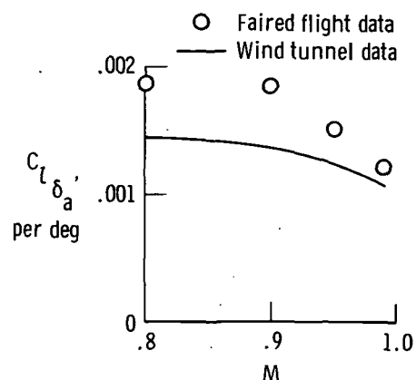
(g) C_{l\delta_a}'
