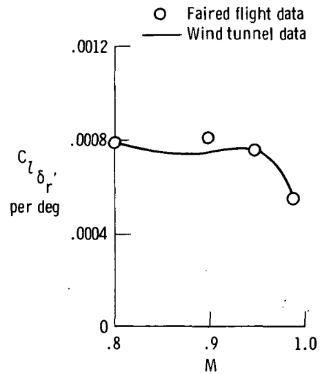
(d) C_{l_{\delta_r}} .
