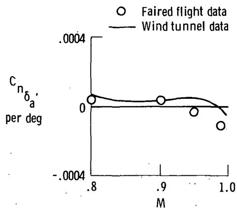
(h) C_{n\delta_a}'
