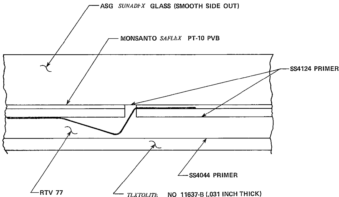
Figure 3-9. Module Encapsulation
