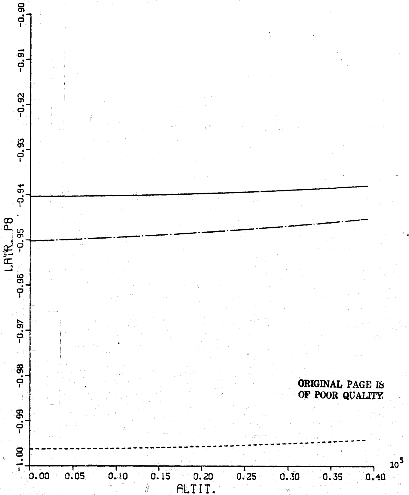
Fig. A.28 LATR. P8 VS. ALTIT. (Liapunov IAS)
