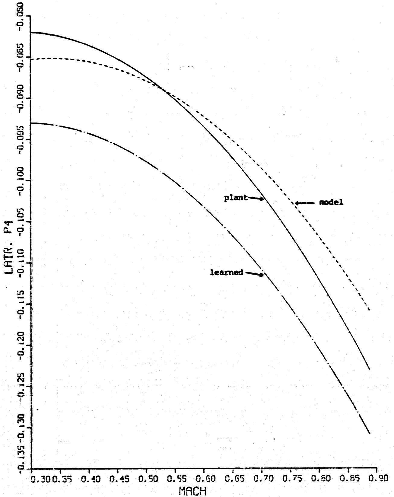
Fig. 4.9 LATR. P4 VS. MACH (Liapunov IAS)
