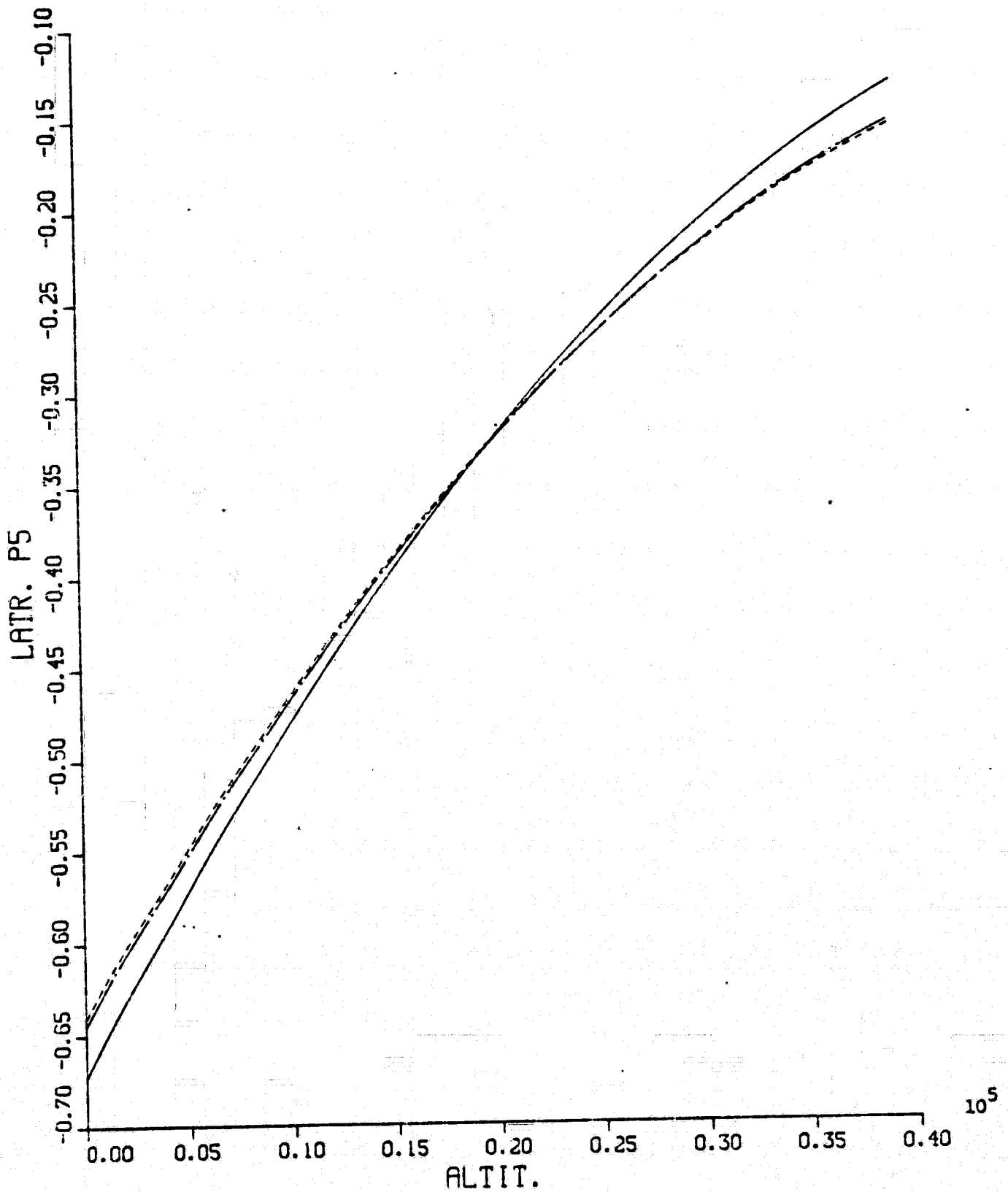
Fig. A.25 LATR. P5 VS. ALTIT. (Liapunov IAS)
