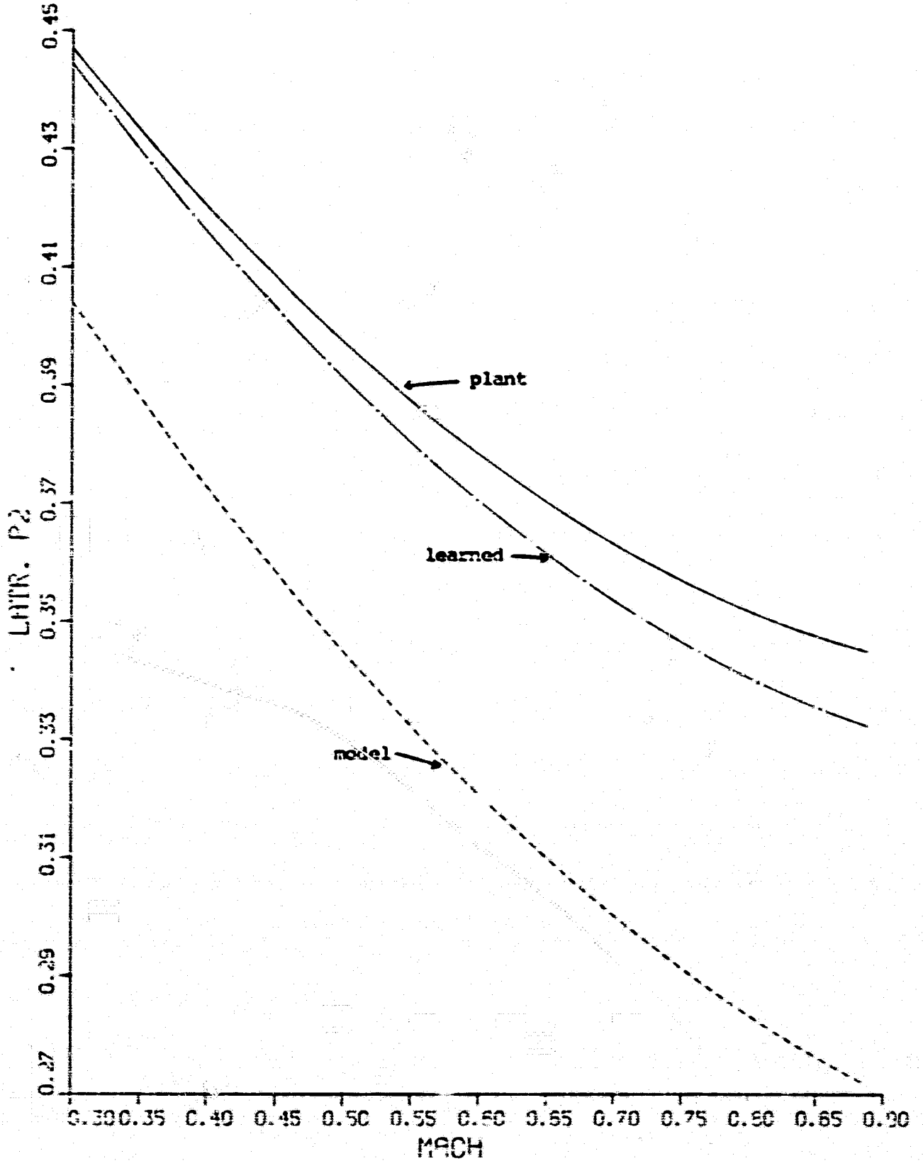
Fig. 4.8 LAIR. P2 VS. MACH (Liapunov IAS)
