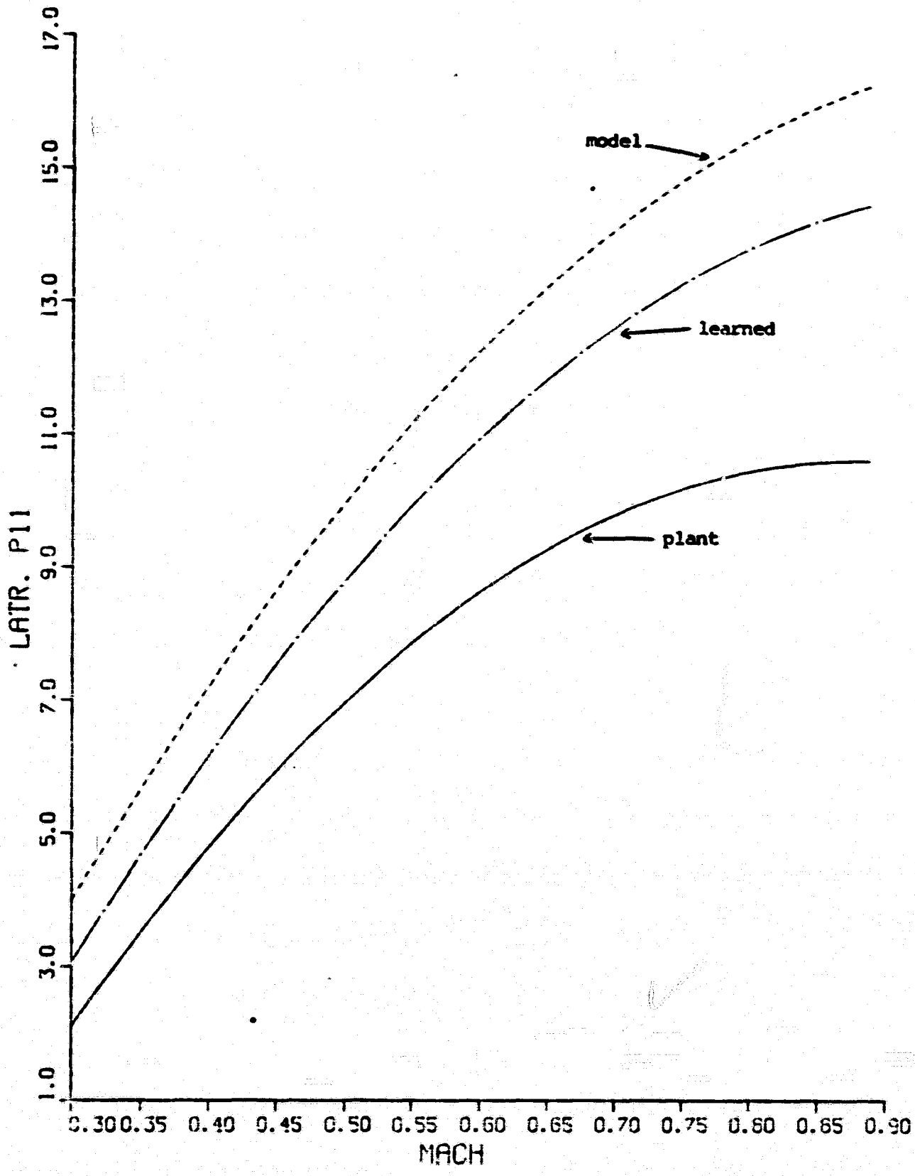
Fig. 4.10 LATR. P11 VS. MACH (Liapunov IAS)
