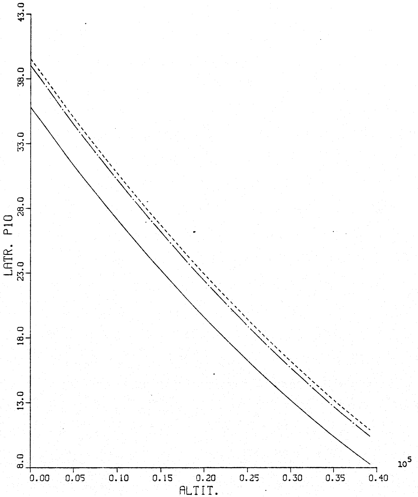
Fig. A.30 LATR. P10 VS. ALTIT. (Liapunov IAS)
