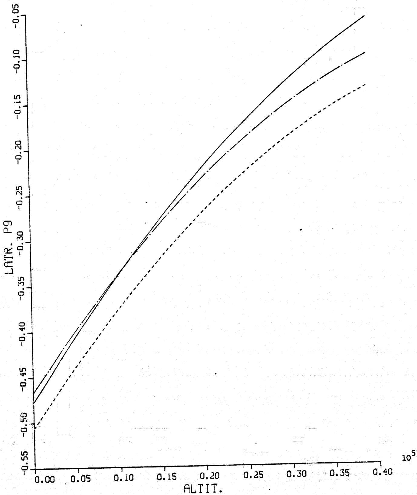
Fig. A.29 LATR. P9 VS. ALTIT. (Liapunov IAS)
