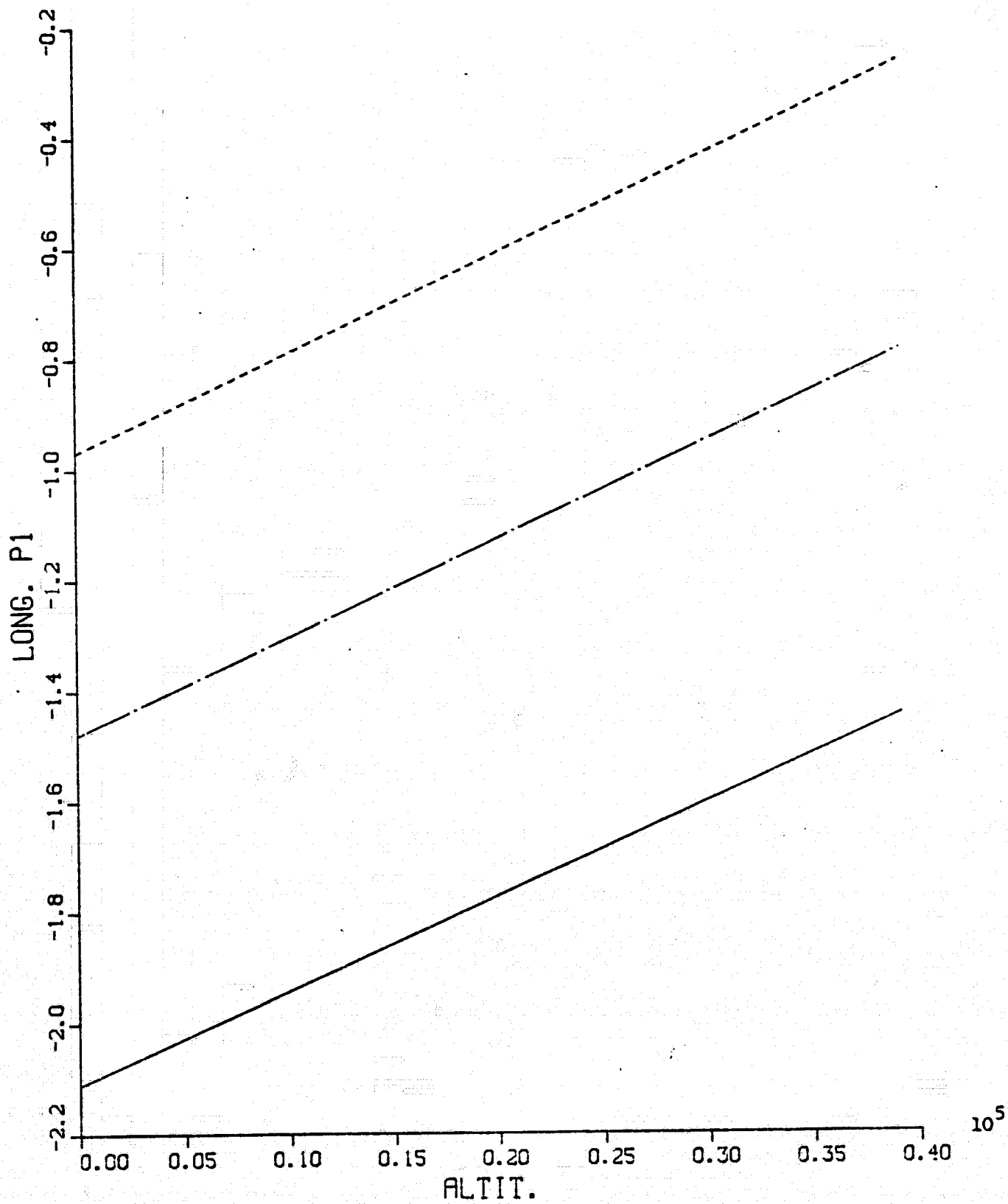
Fig. A.1 LONG. P1 VS. ALTIT. (Liapunov IAS)
