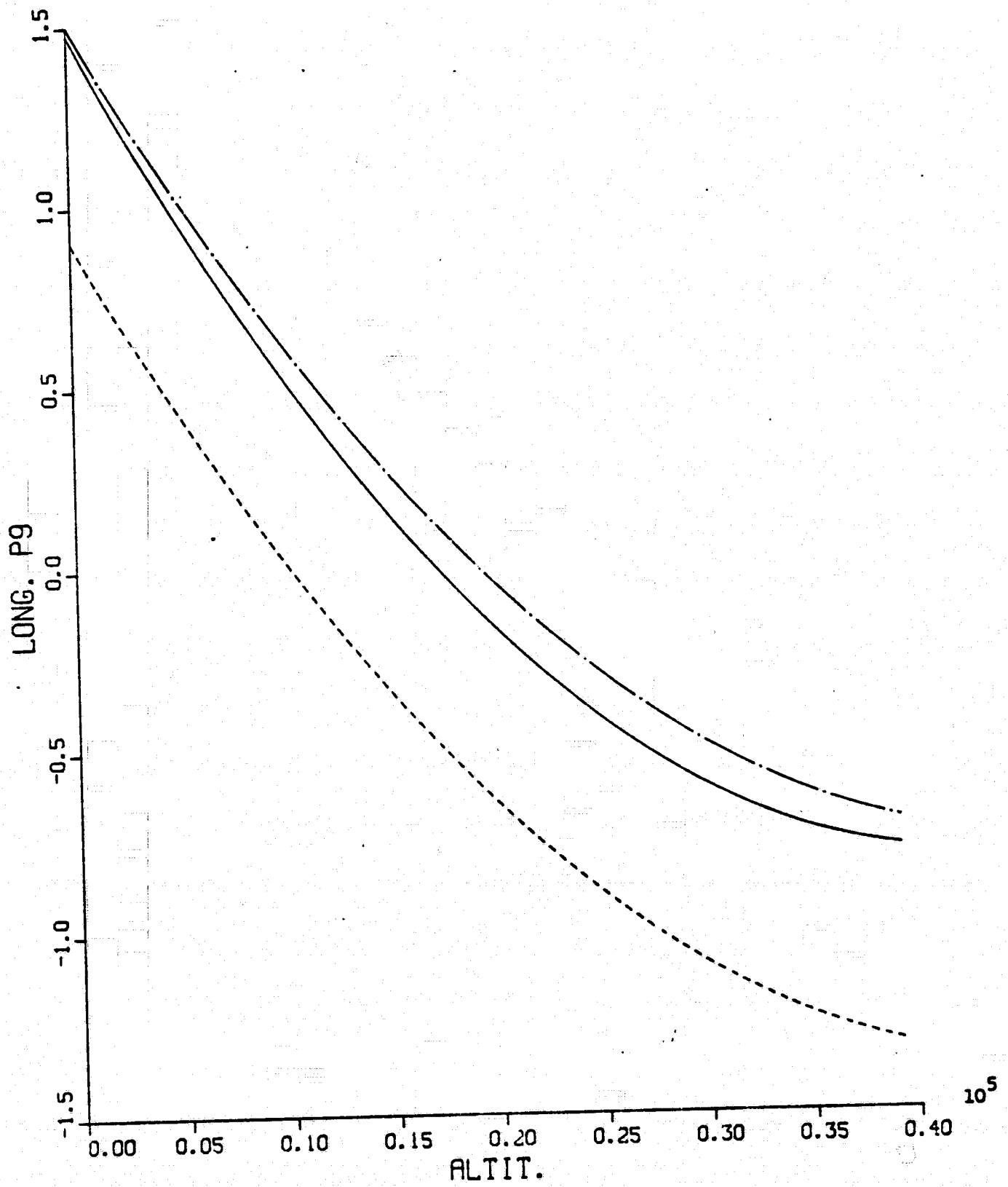
Fig. A.9 LONG. P9 VS. ALTIT. (Liapunov IAS)
