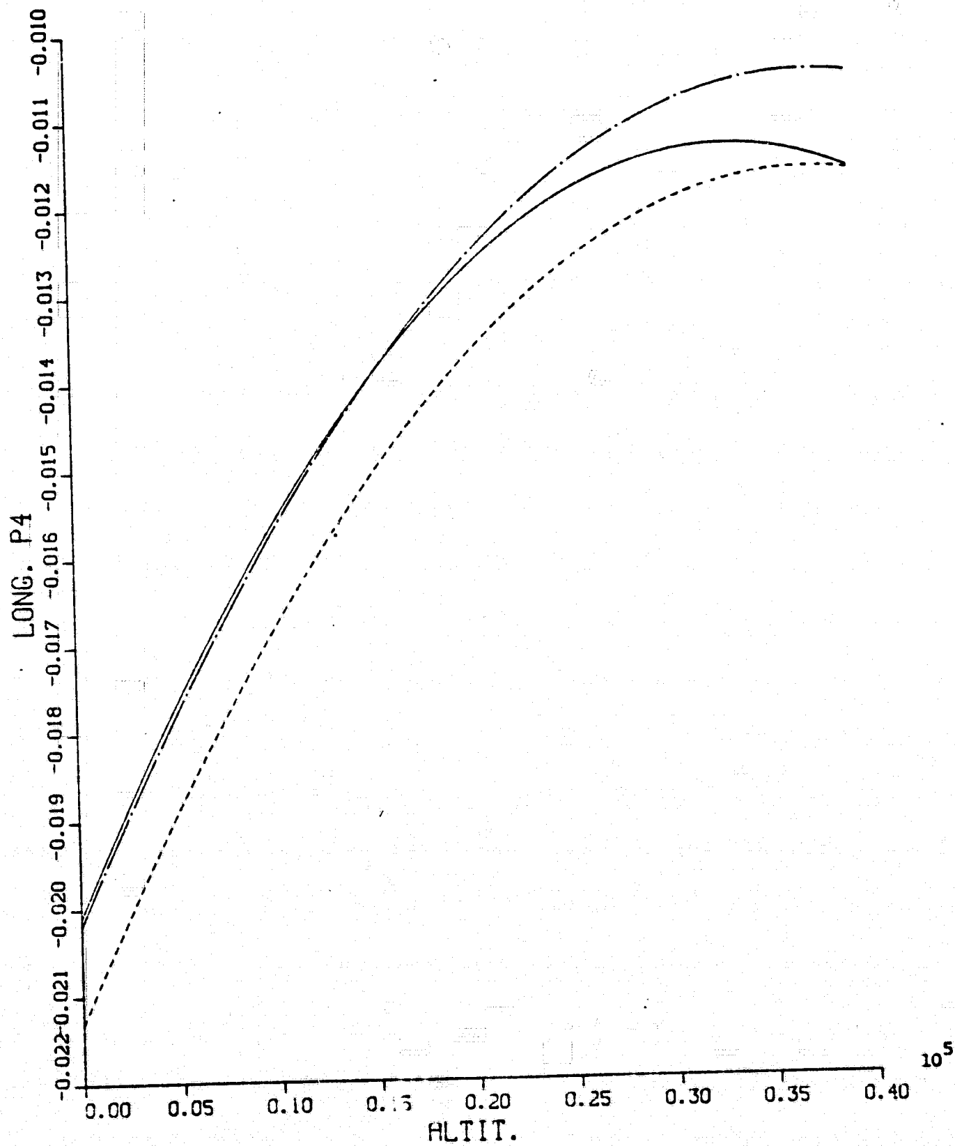
Fig. A.4 LONG. P4 VS. ALTIT. (Liapunov IAS)
