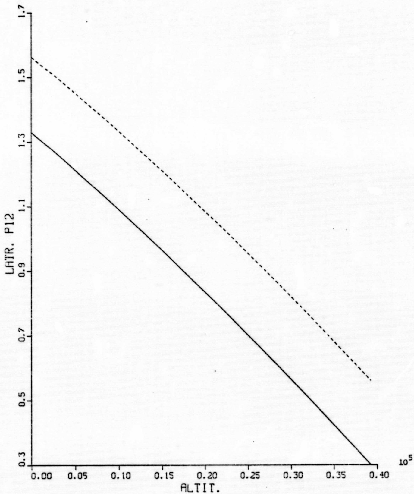
Fig. A.46 LATR. P12 VS. ALTIT. (Newton-Raphson IAS)
