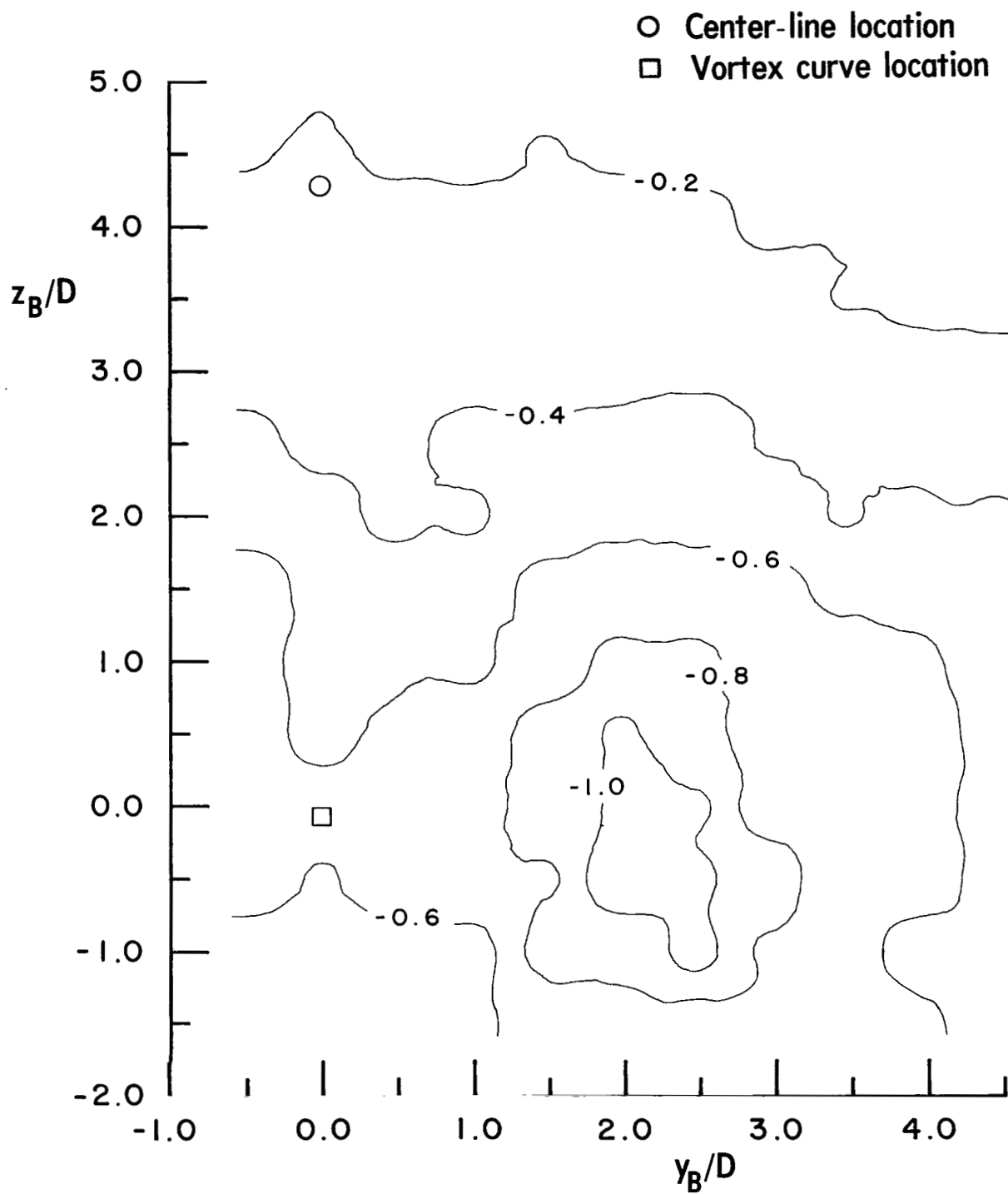
(d) Static-pressure coefficient C_p .
