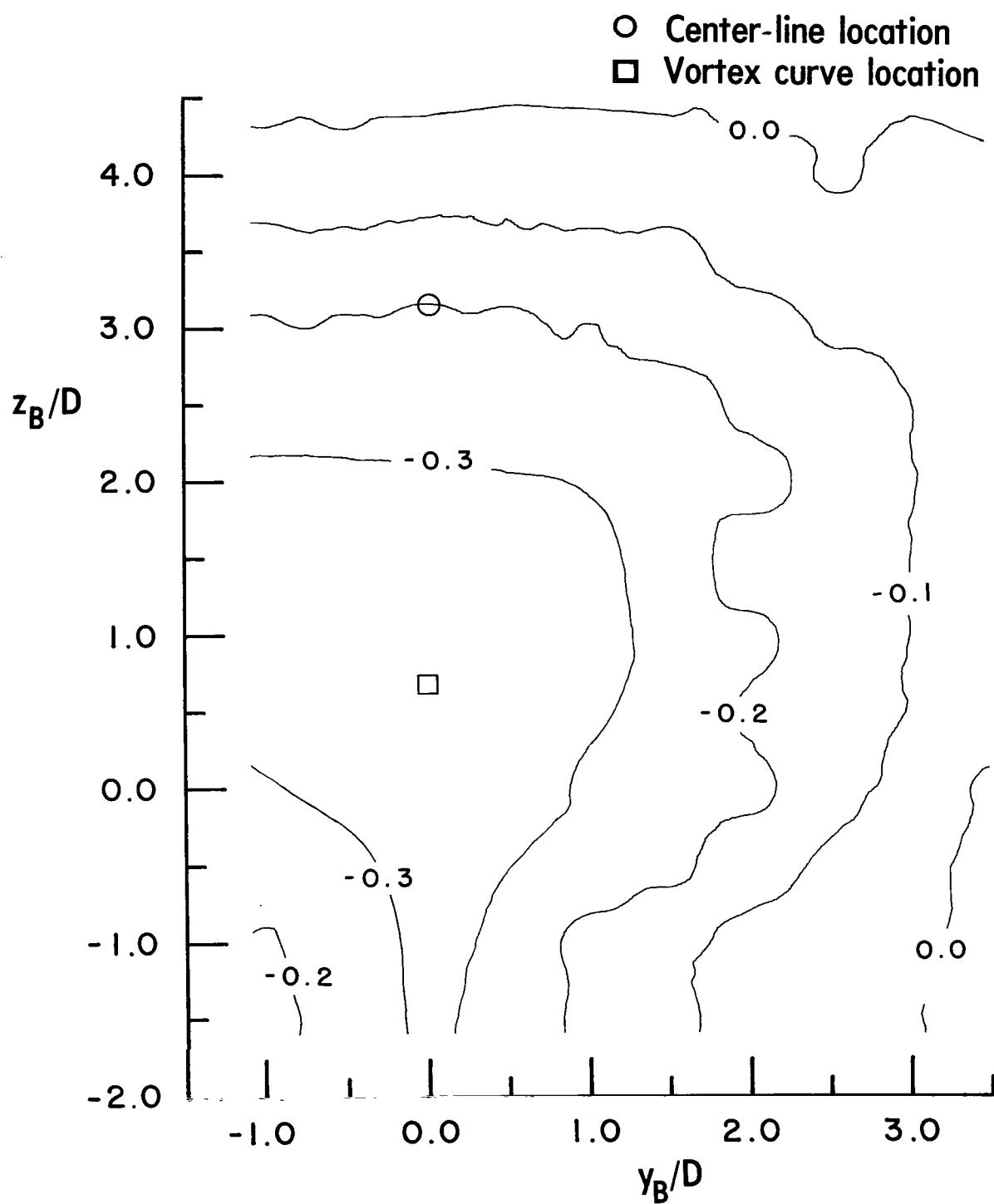
(d) Static-pressure coefficient C_p .
