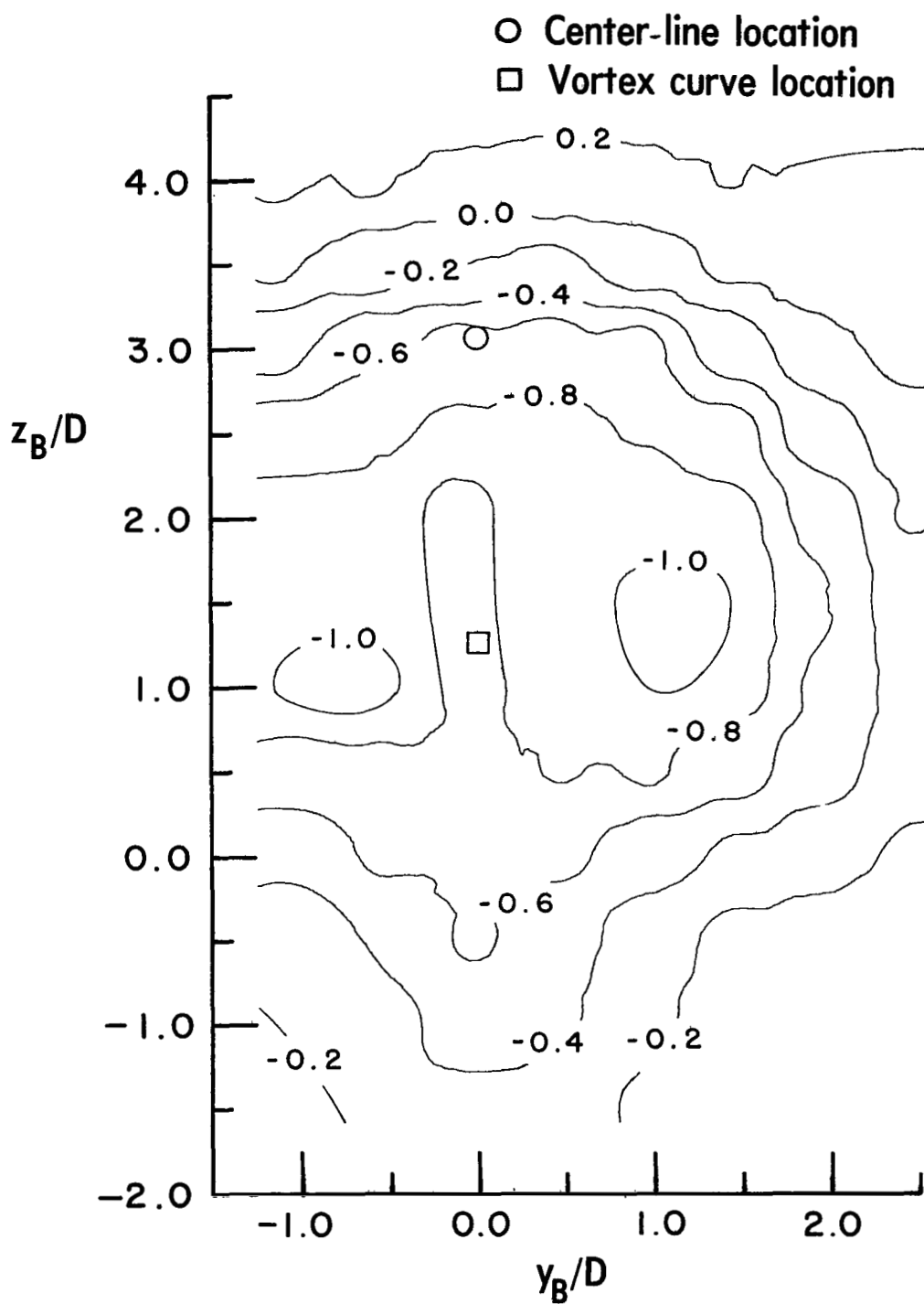
(d) Static-pressure coefficient C_p .
