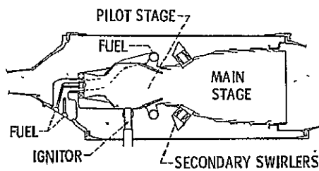
(b) Vorbix combustor.
