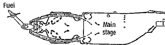
(d) Staged-premixed combustor.
