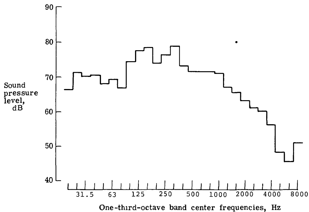
(d) DC-10.
