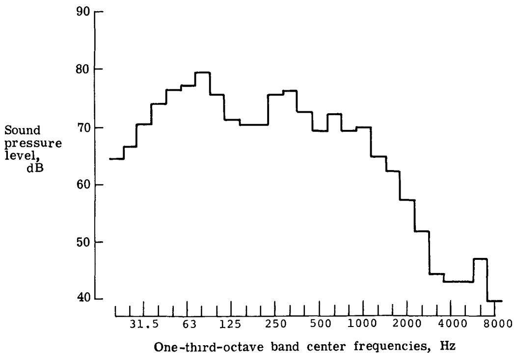
(b) B-727.
