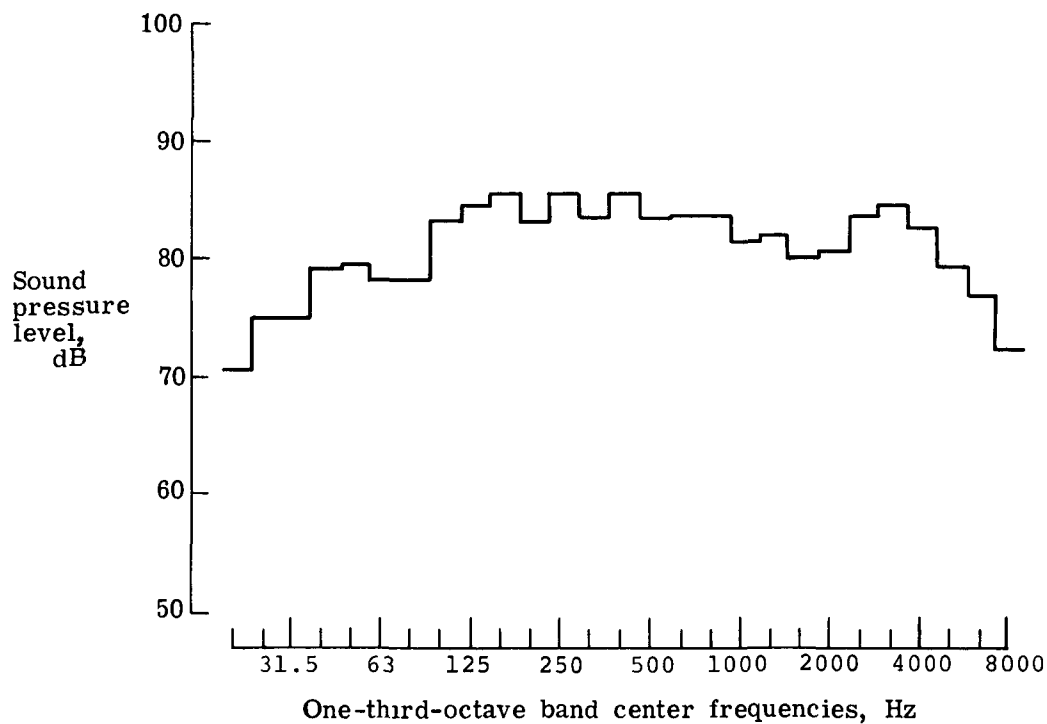
(b) B-727.
