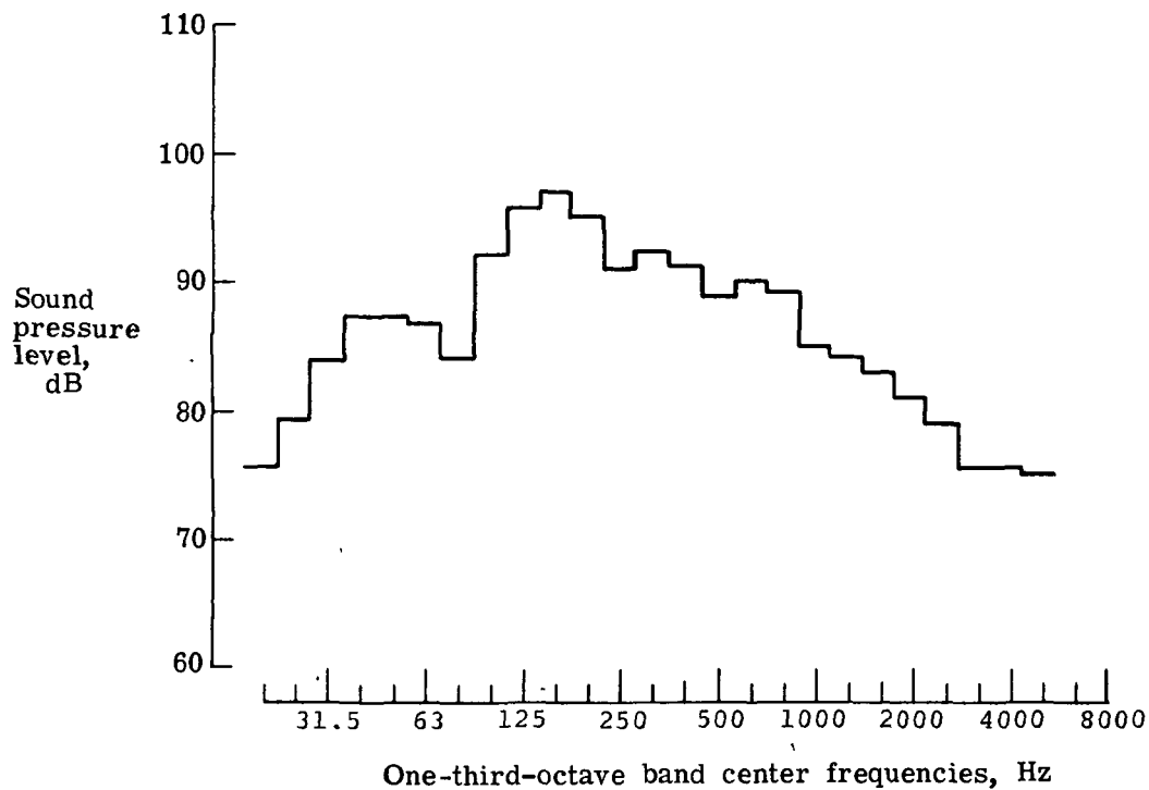
(b) B-727.
