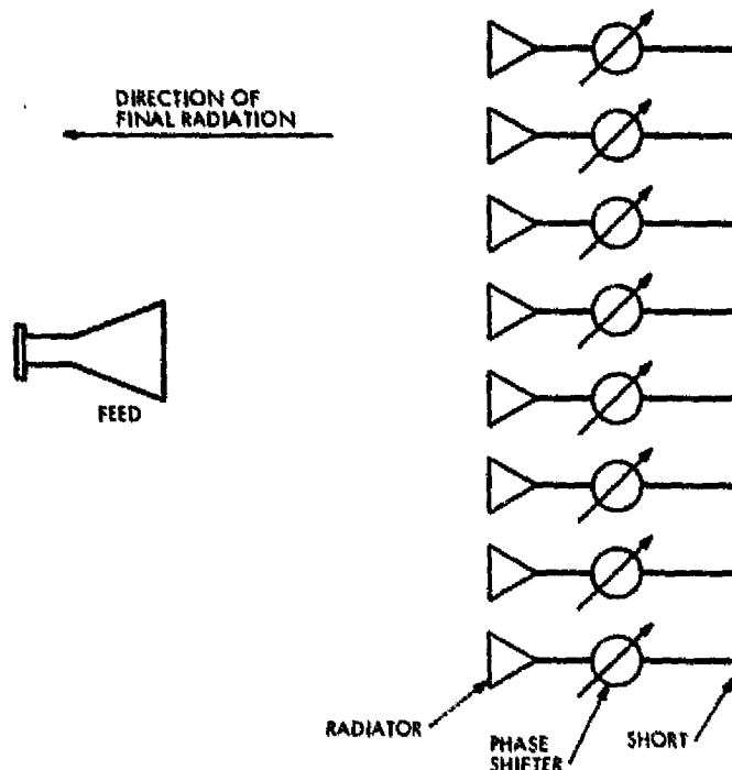
Figure 39. Reflectarray
