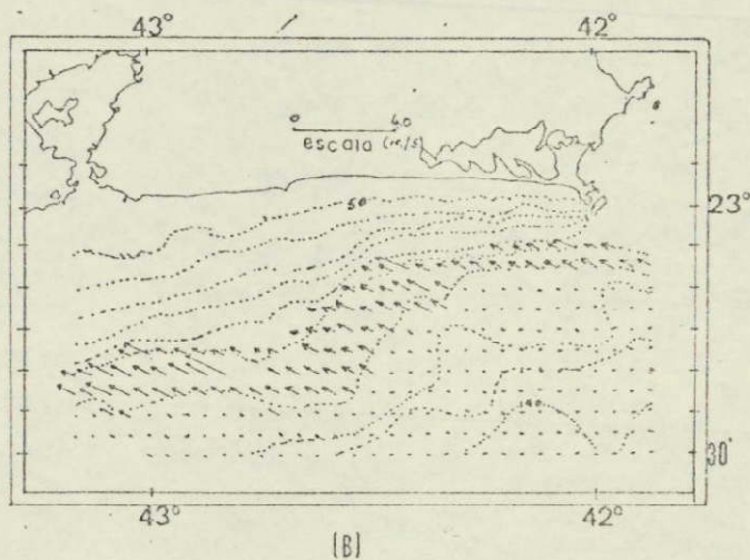
Fig. 6 - (A) e (B) - Campos das Velocidades Horizontais Simulados em m/s na superfície e a 90 metros de profundidade, respectivamente (Tanaka, 1977)
