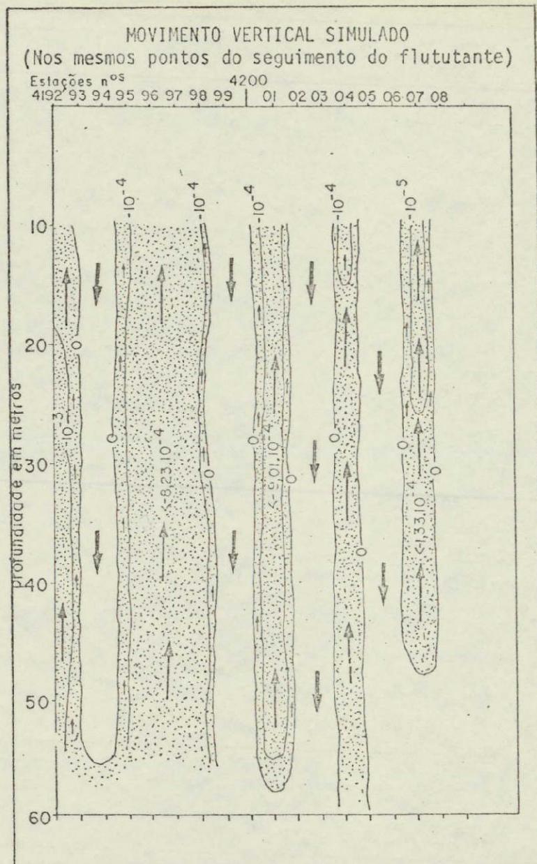
Fig. 3 - Movimento Vertical Simulado em m/s
