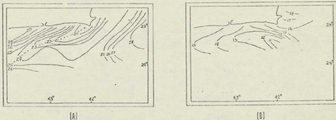
Fig. 7 - (A) e (B) - Distribuição da temperatura, em ^{\circ}\text{C} na superfície e no fundo, respectivamente, em condições de ressurgência (Rodrigues, 1977)
