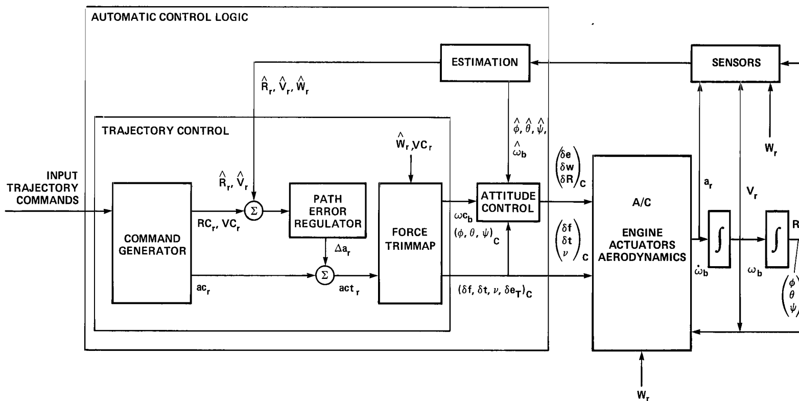
Figure 1.- Automatic control logic - AWJSRA.
