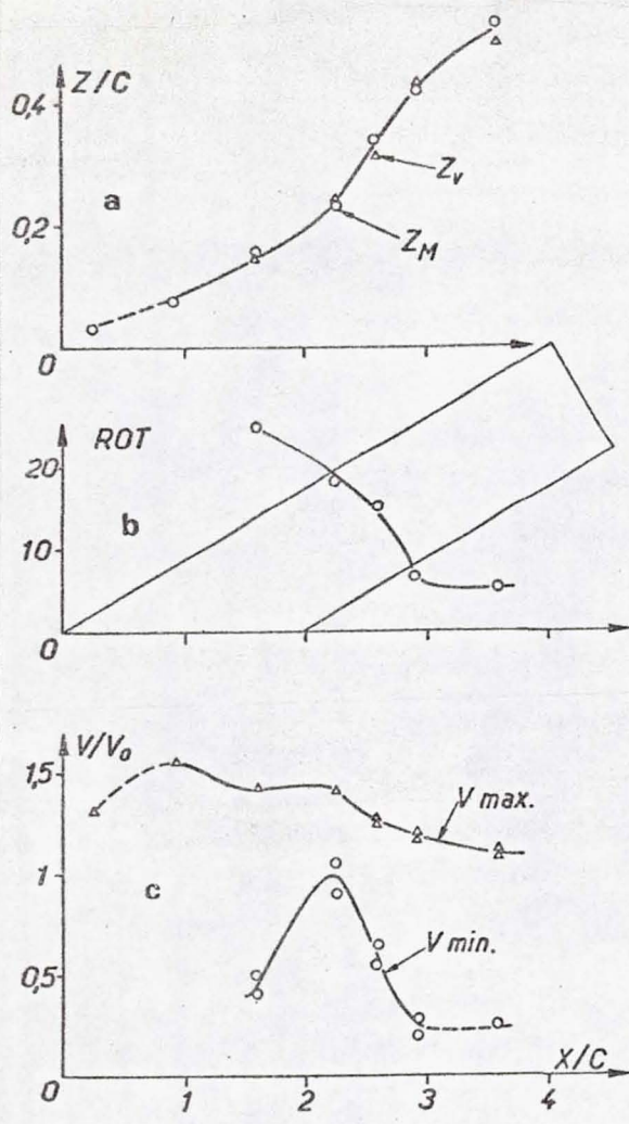
Fig. 25 - Longitudinal Evolution of the Vortex
