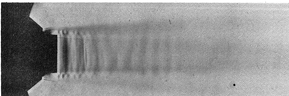
(f) \xi_p = 1.853
