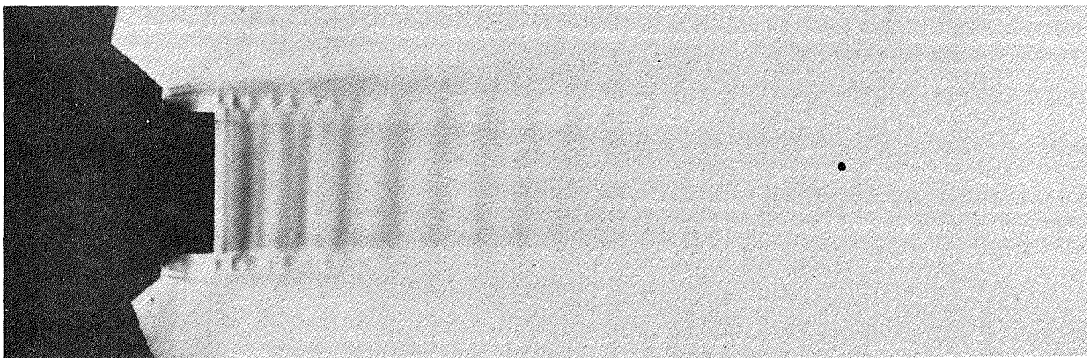
(d) \xi_p = 1.776
