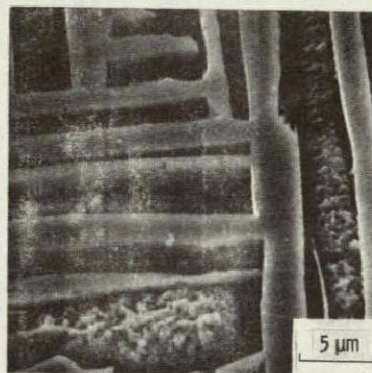
LAMELLAR \text{Ni}_3\text{Cb} ; \gamma/\gamma'-\delta CS-76751
