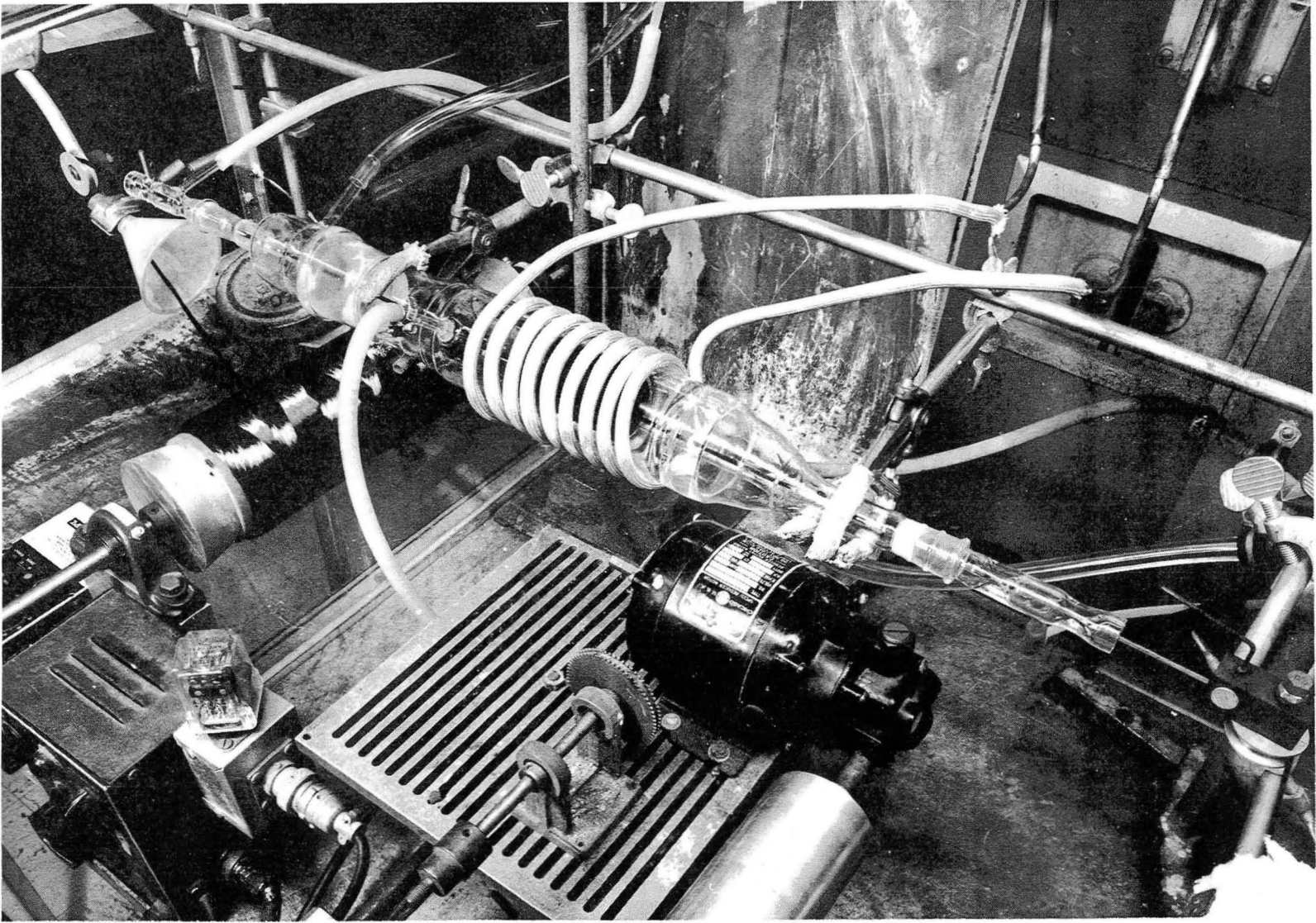
Fig. 5 Horizontal CVD SiC Apparatus
