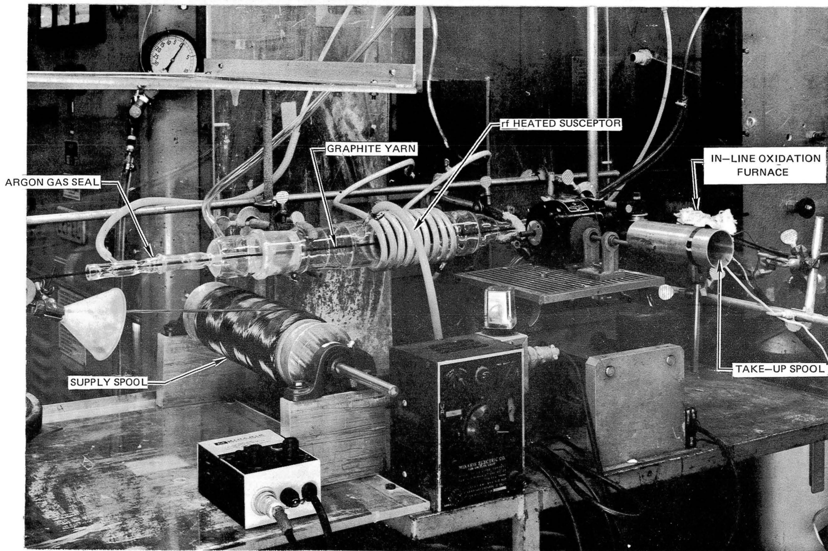
Fig. 4 Horizontal CVD SiC Apparatus
