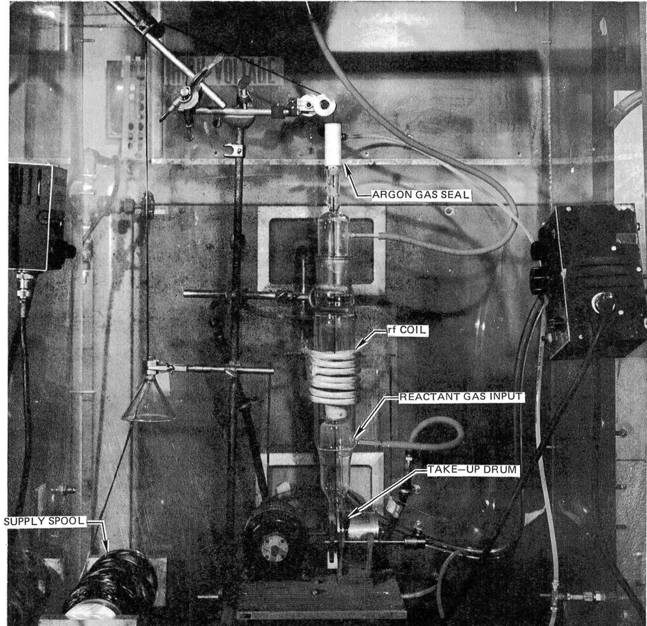
Fig. 3 Vertical CVD SiC Apparatus
