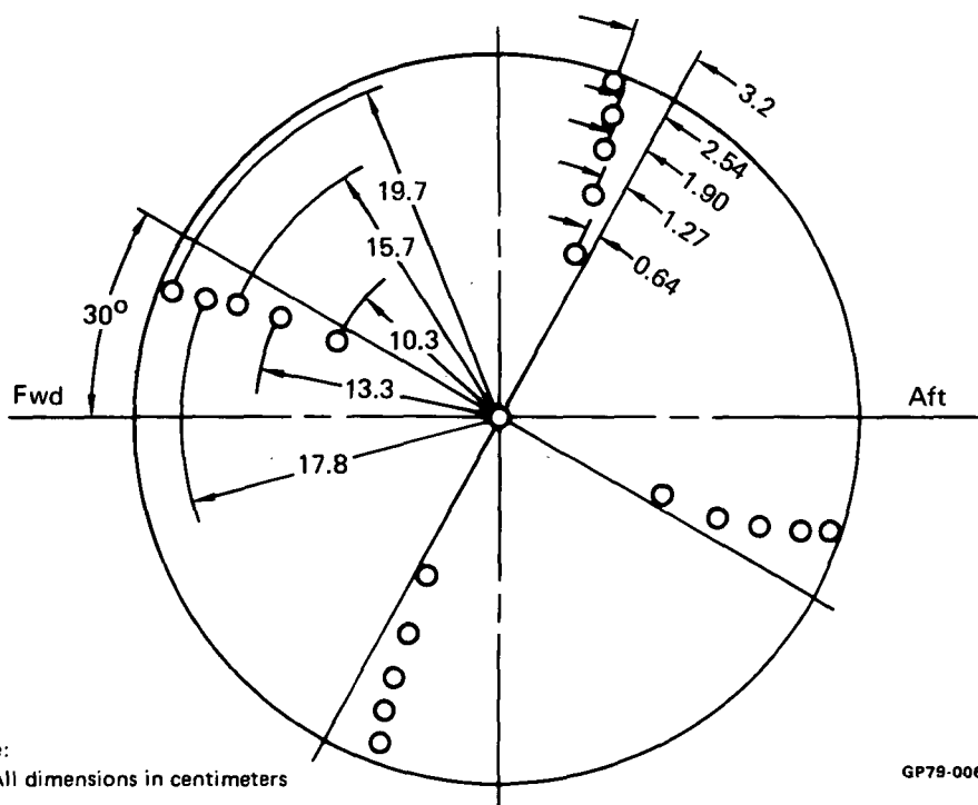
Section A-A
