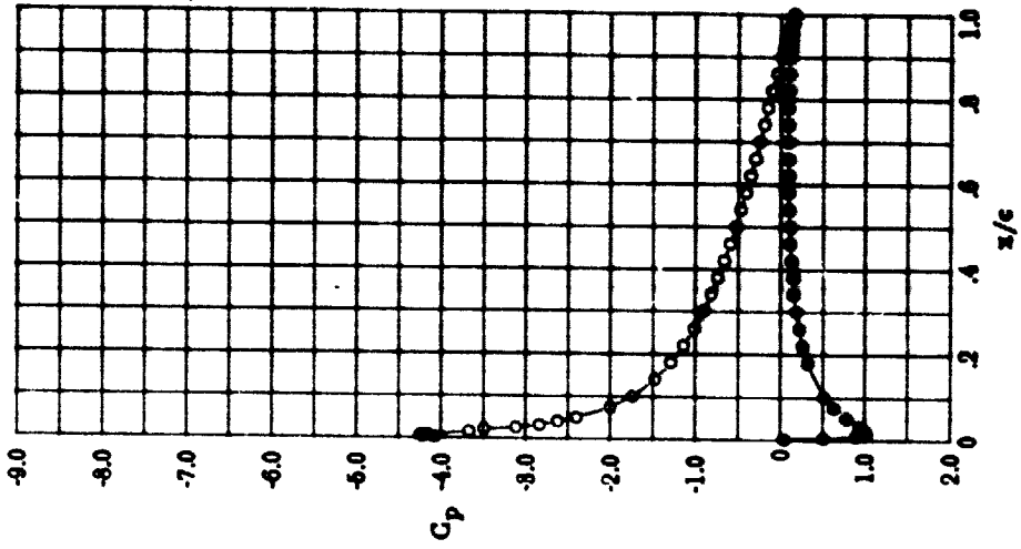
(h) M=3.01 ; c_e=.959 ; \alpha=9.96
