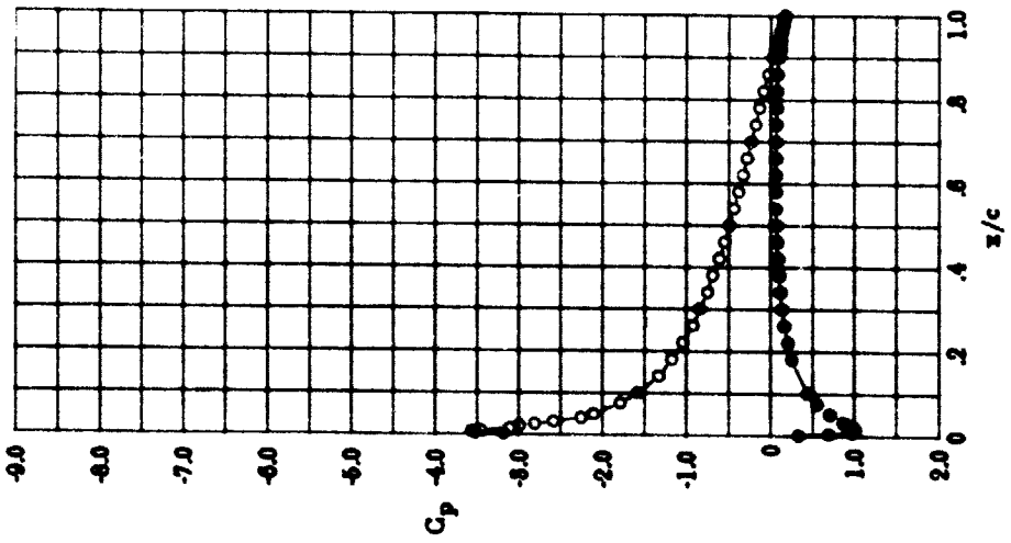
(g) M=3.00 ; c_e=.849 ; \alpha=8.86
