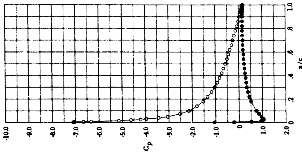
(d) M=301 ; c_a=1.220 ; \alpha=12.88
