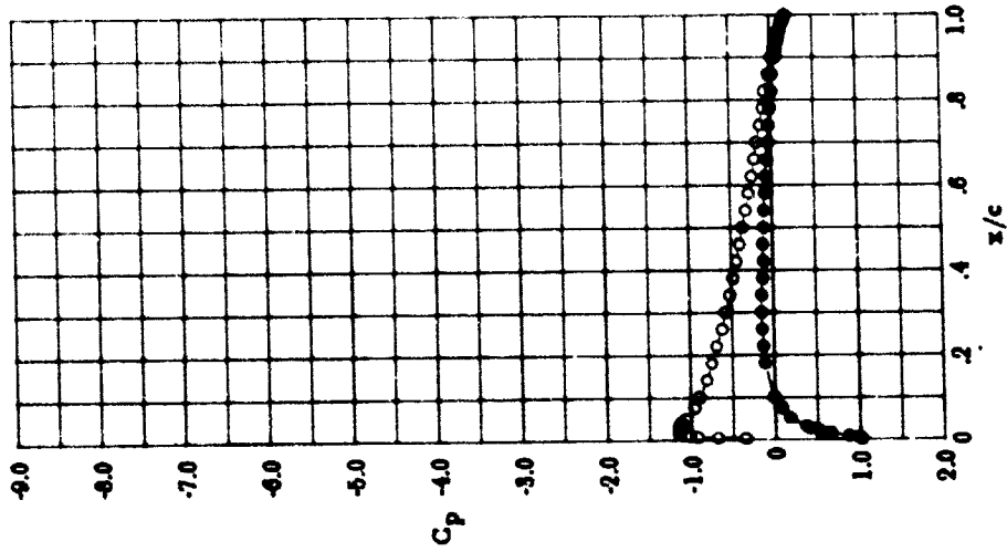
(d) M=0.303 ; c_u = 0.376 ; \alpha = 3.66
