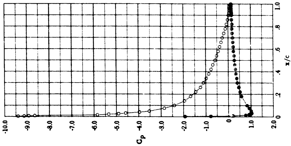
(f) M=300 ; c_a=1.356 ; \alpha=14.88
