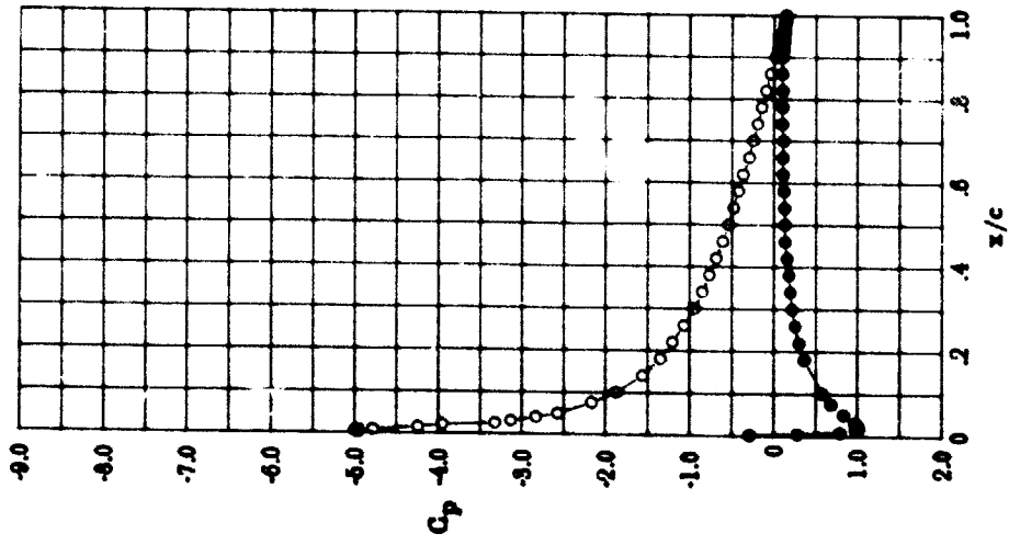
(i) M=2.99 ; c_e=1.026 ; \alpha=10.86
