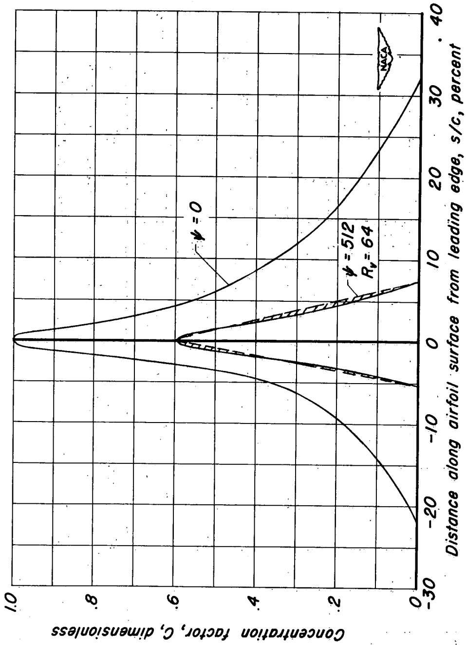
(d) 15-percent-thick cambered Joukowski airfoil; a = 1.0 mean line; \alpha = 0^\circ .
