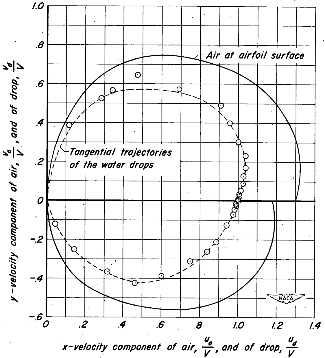
(d) 15-percent-thick cambered Joukowski airfoil; a = 1.0 ; \alpha = 0^\circ .
