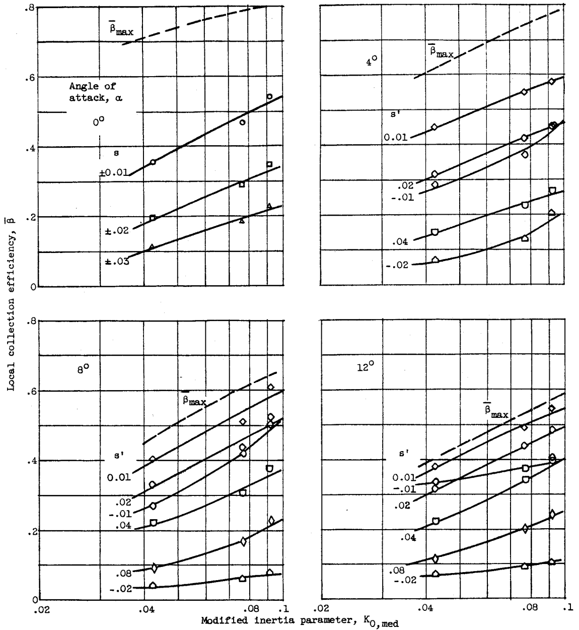
(d) NACA 65 2 -015 airfoil. Chord, 13 inches.
