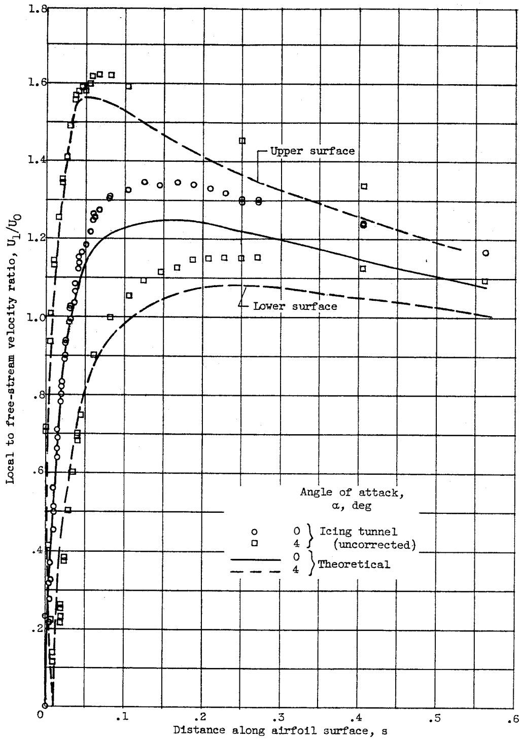
(a) Joukowski 0015 airfoil; 96-inch chord.
