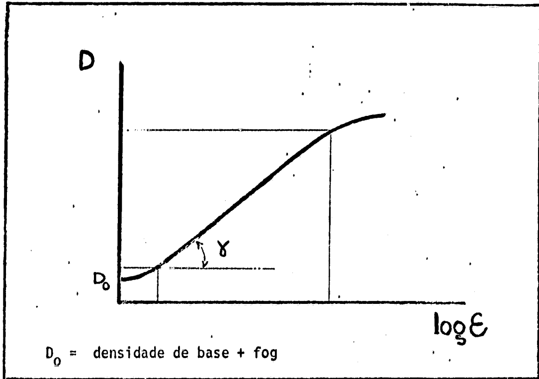
Fig. 2.4 - Curva característica de um filme P&B.
