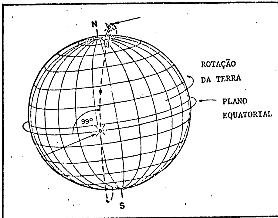
Fig. 3.3 - Órbita do satélite LANDSAT.
