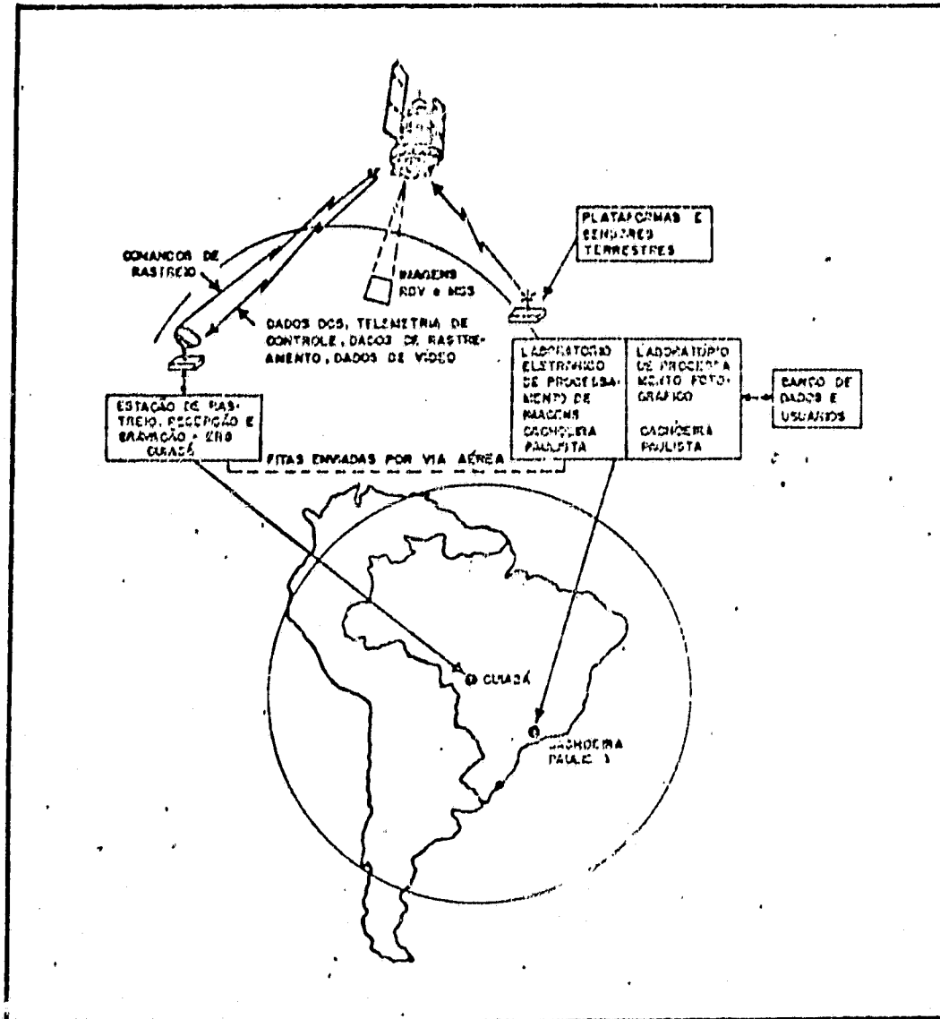
Fig. 3.1 - Configuração do Sistema LANDSAT, utilizada pelo Instituto de Pesquisas Espaciais - INPE.
