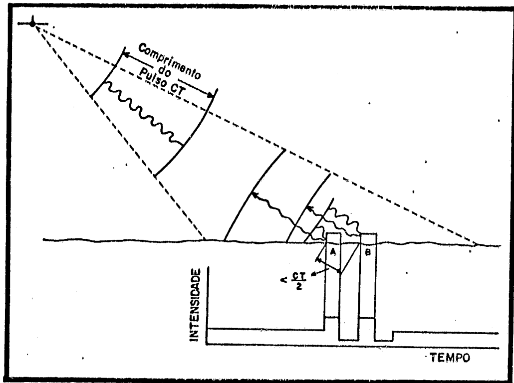
Fig. 2.10 - Radar de Visada Lateral.
