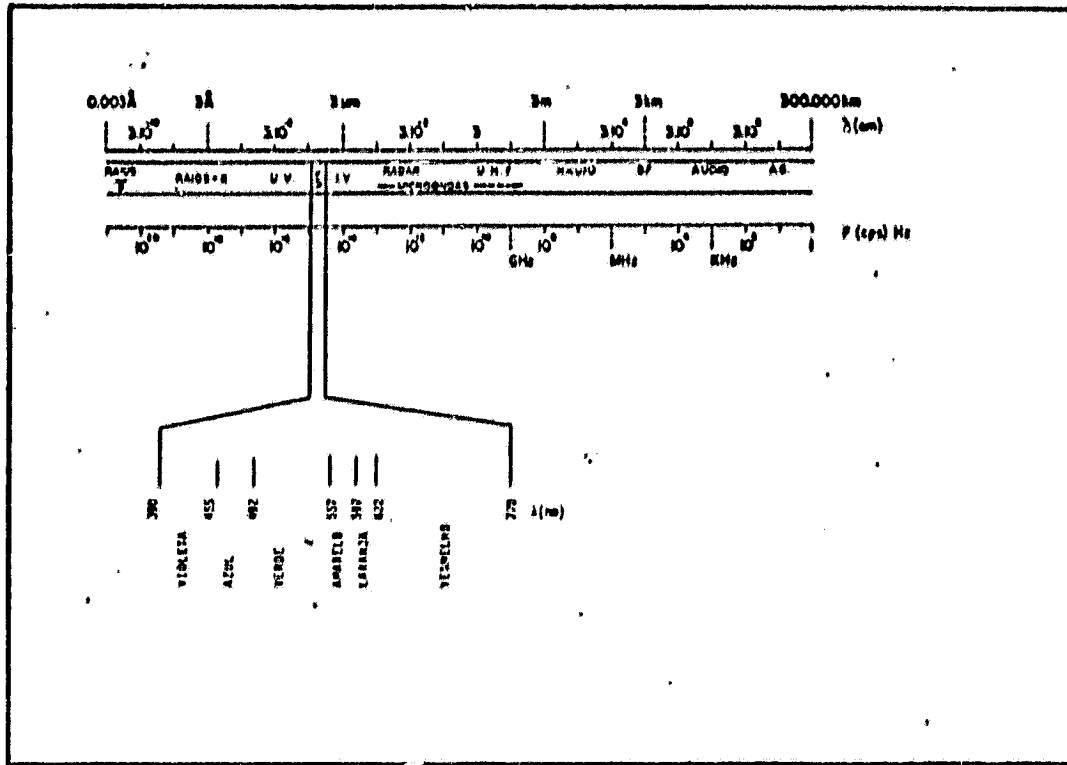
Fig. 1.2 - Espectro Eletromagnético.
