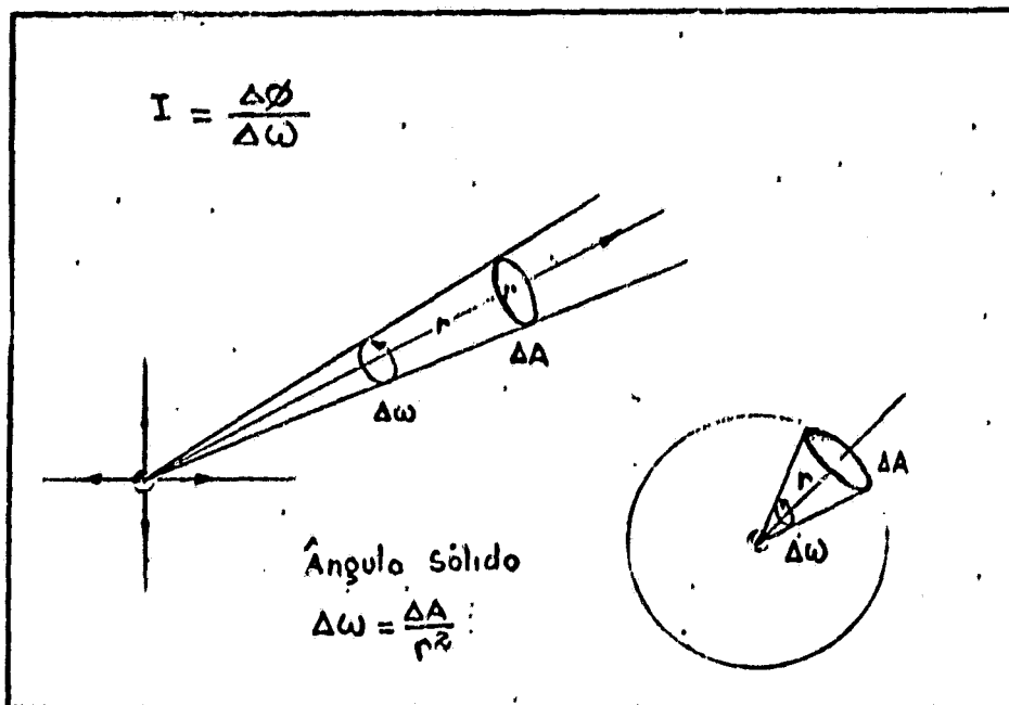
Fig. 1.3 - Intensidade radiante e ângulo sólido.
