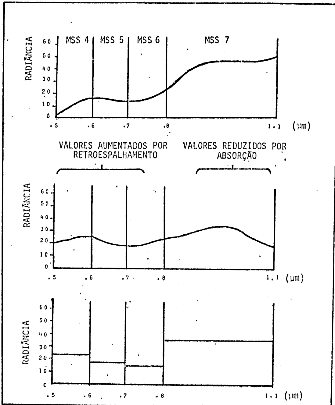
Fig. 3.13 - Influência atmosférica na aquisição dos dados MSS-LANDSAT.
