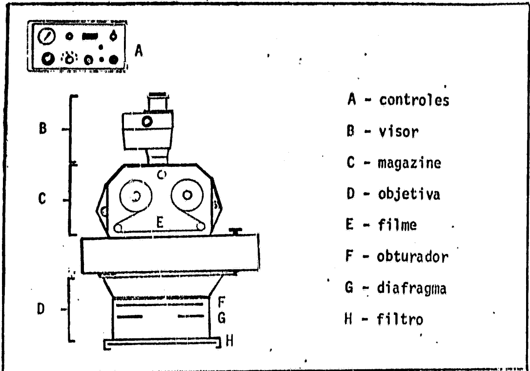
Fig. 2.3 - Partes de uma câmara fotográfica aérea.
