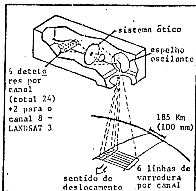
Fig. 3.6 - Sistema imageador MSS-LANDSAT.
