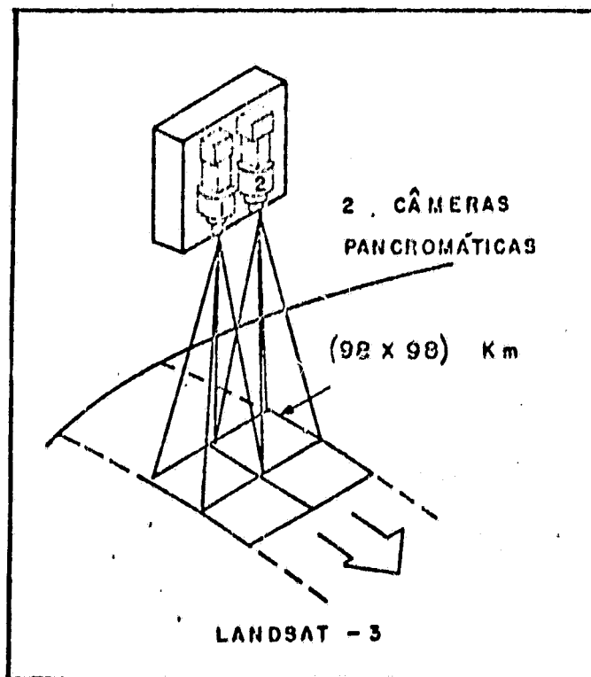
Fig. 3.10 - Configuração do Sistema RBV - LANDSAT 3.
