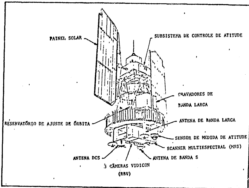
Fig. 3.2 - Configuração do satélite LANDSAT.
