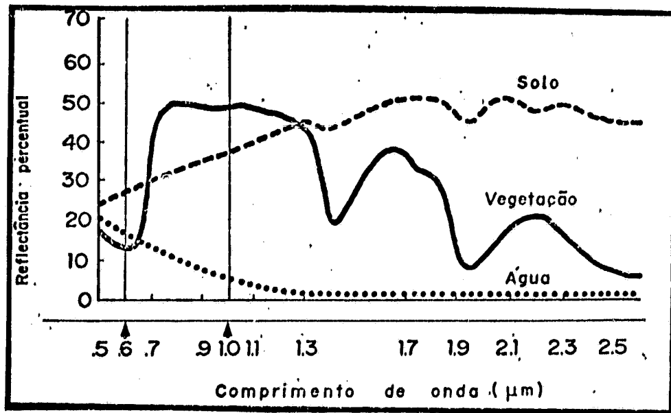
Fig. 1.6 - Reflectância espectral de amostras de solo, de água e de vegetação.
