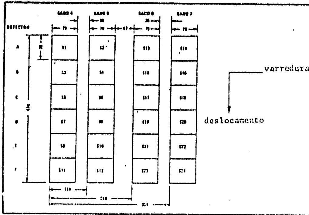
Fig. 3.7 - Geometria da matriz de terminais de fibras ópticas do MSS -LANDSAT 1 e 2.
