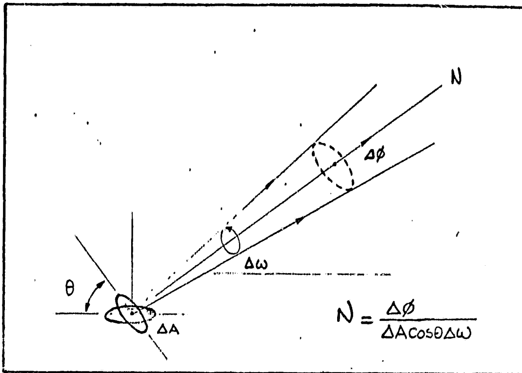
Fig. 1.4 - Radiância de uma superfície
