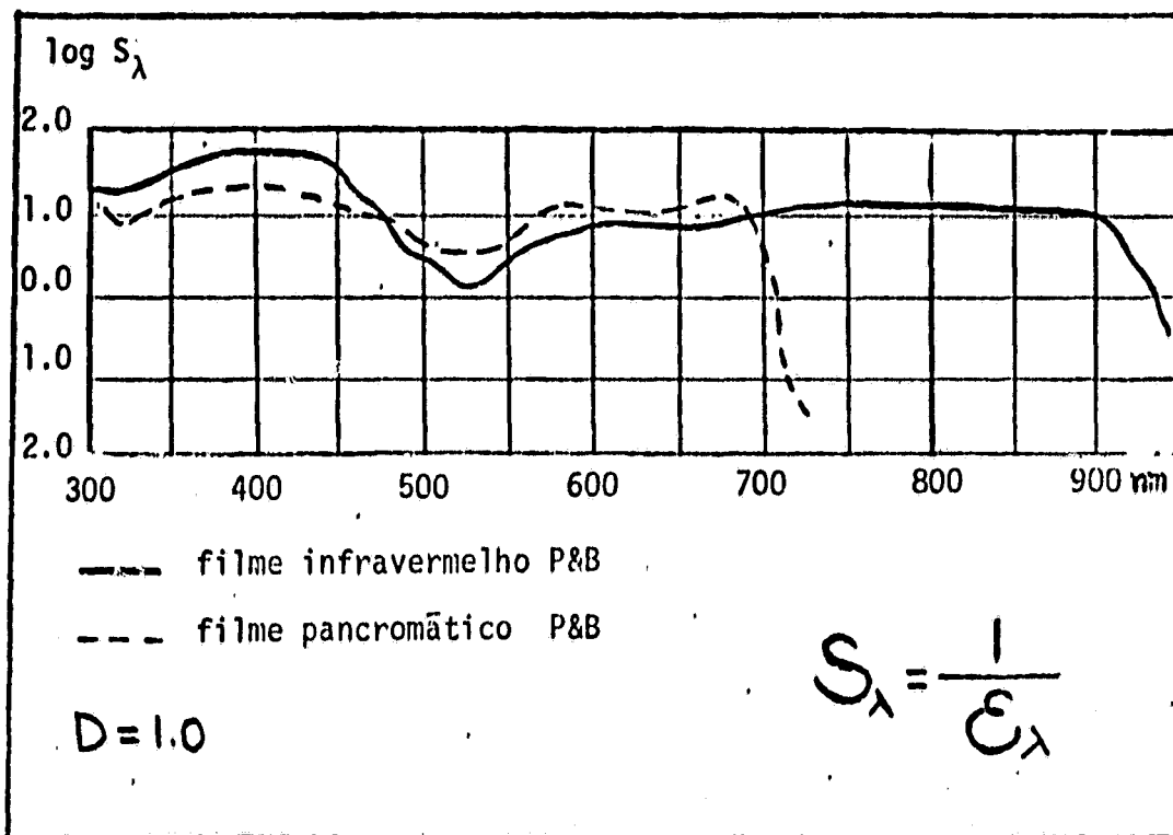
Fig. 2.5 - Sensitividade espectral.
