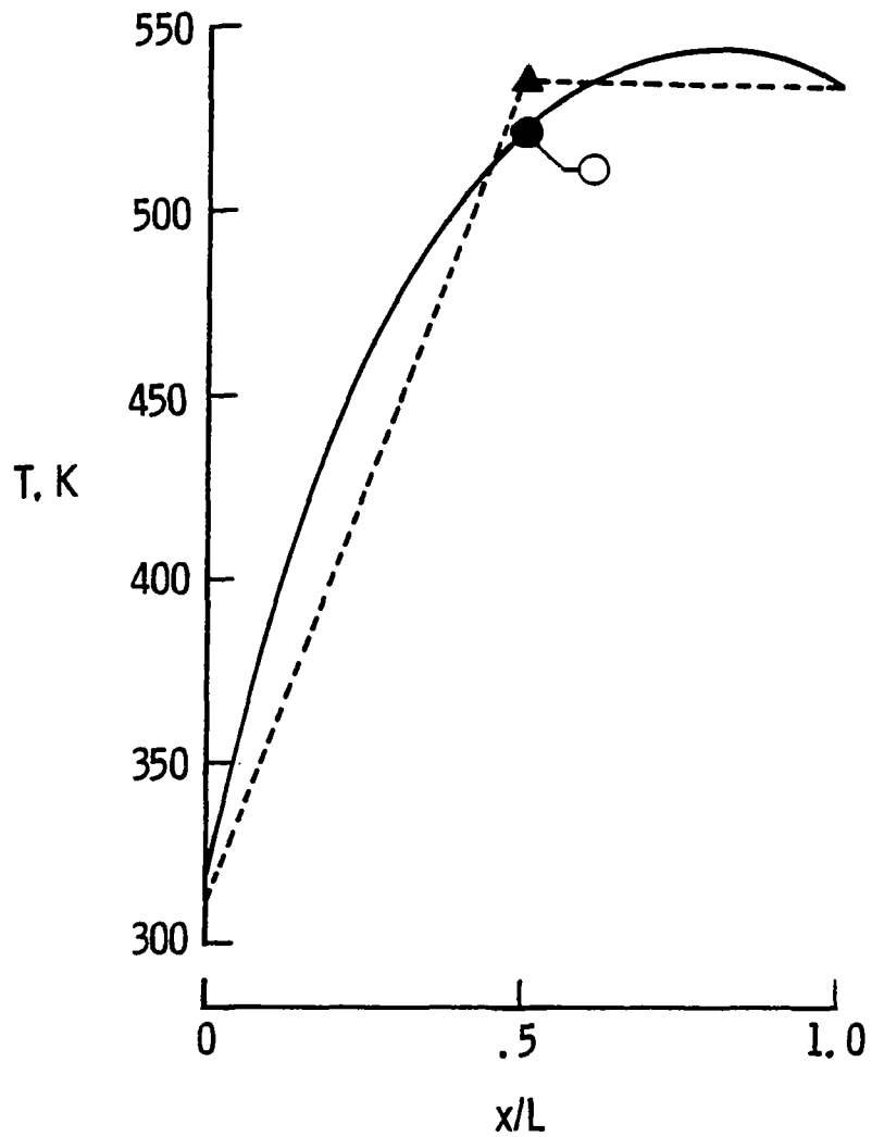
(d) Comparative temperature distributions at t = .30 s.
