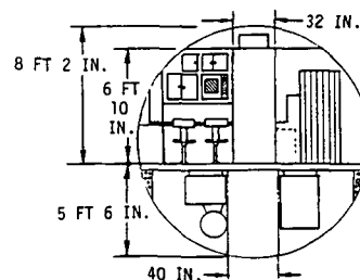
ENERGY MODULE - 20 ft LONG
