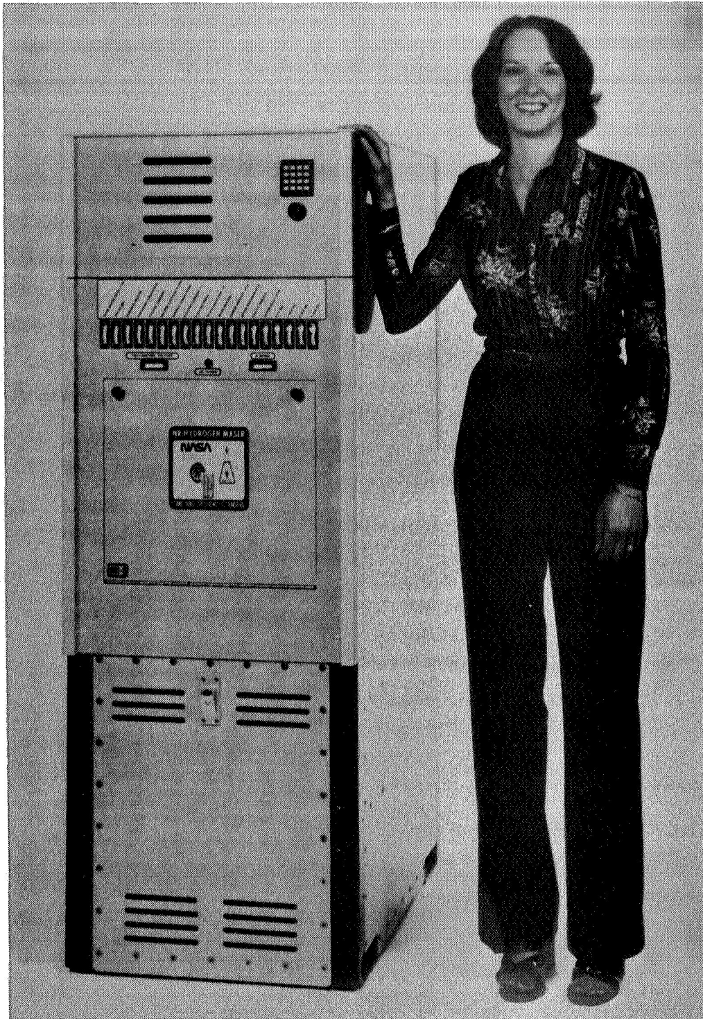
Figure 12. NR Maser
