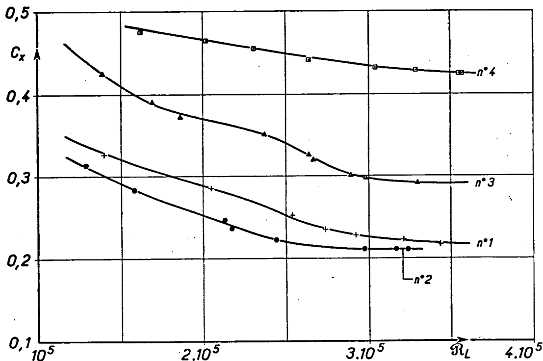
Fig. 12 — AGARD B : M = 5,3 n° 1 + \rho/R = 0 , x = 0 . n° 2 \bullet \rho/R = 0,117 , x = 1 . n° 3 \Delta \rho/R = 0,34 , x = 3 . n° 4 \square \rho/R = 0,624 , x = 6 .
