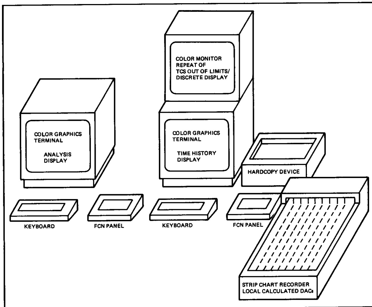
Fig. 4 DAS Hardware
