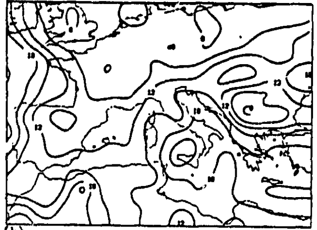
(b) PREC. WATER ABOVE 1000MB(CH#10) 5 MAR 1982 03Z SAT
