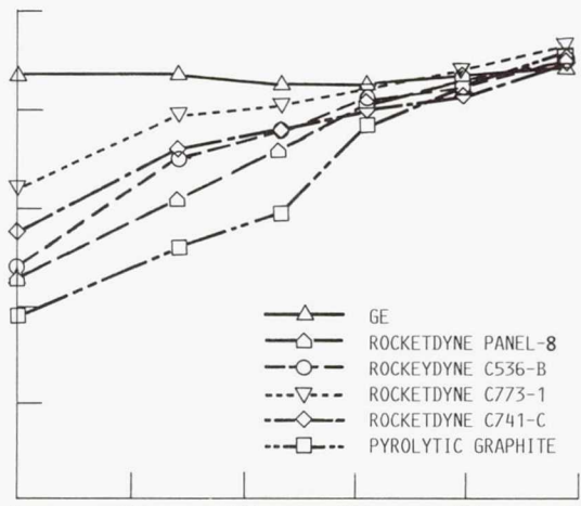
(d) BATCH 2, TOTAL THERMAL EMITTANCE AT 800 K.
