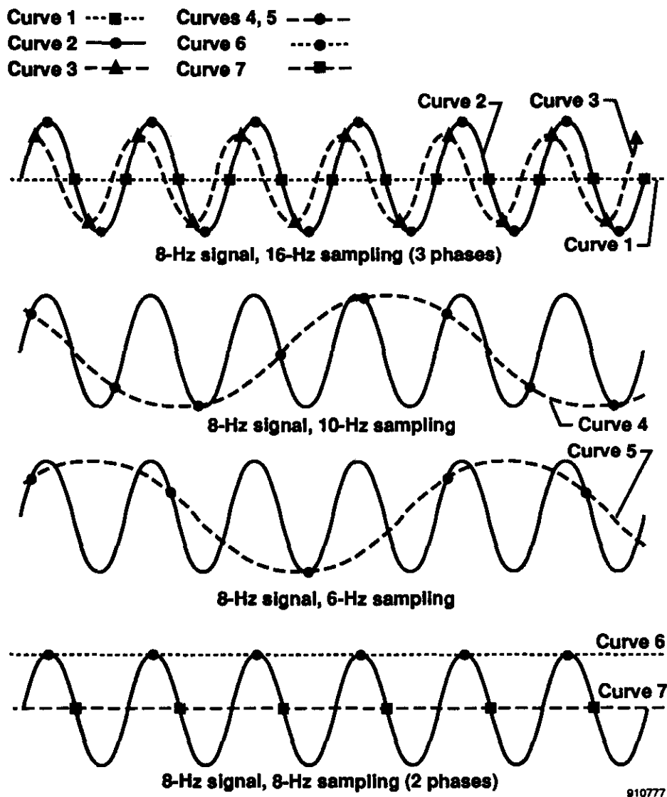
Figure 3-8. Sampling data.
