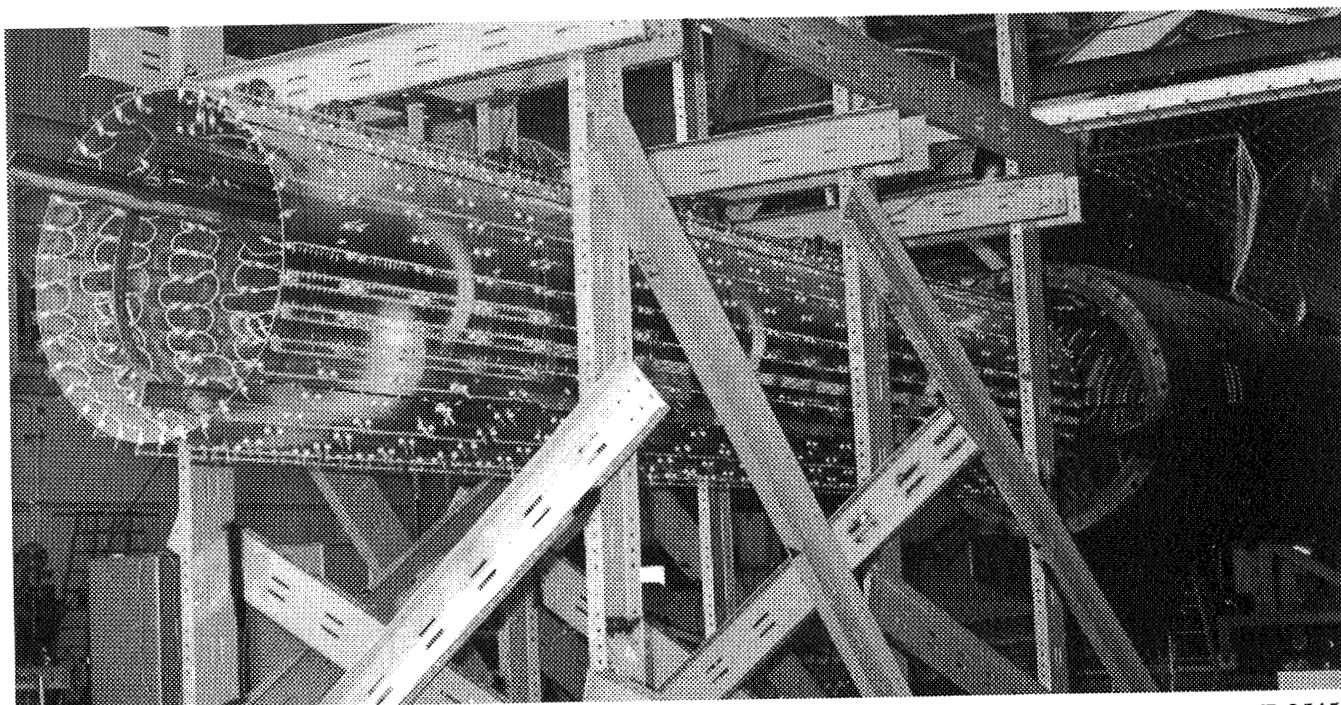
Fig. 34: Internal nacelle heater
