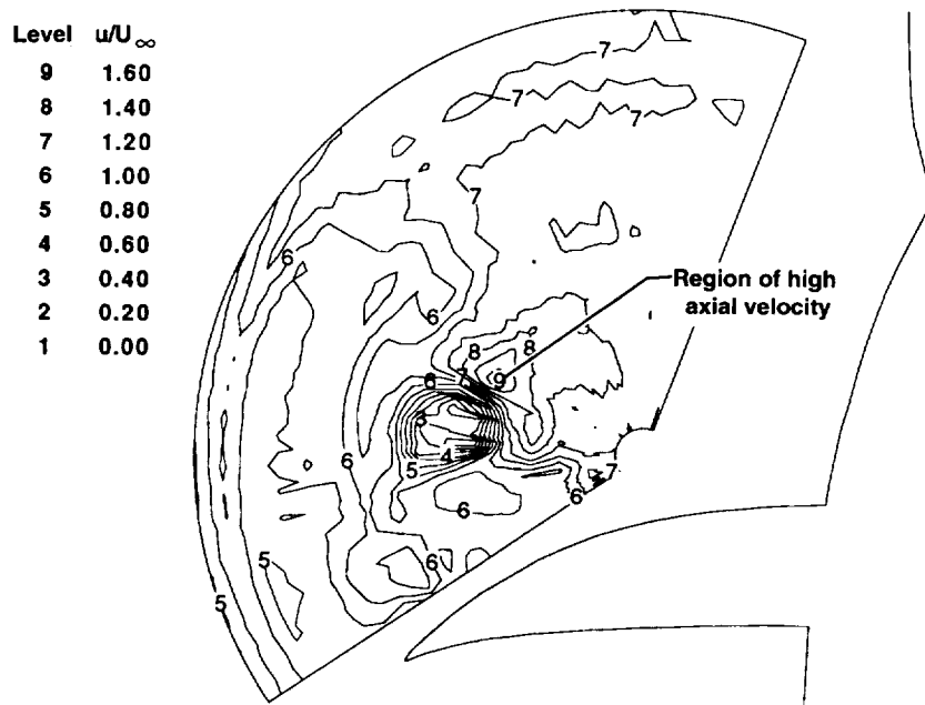
(d) Normalized axial velocity contours.
