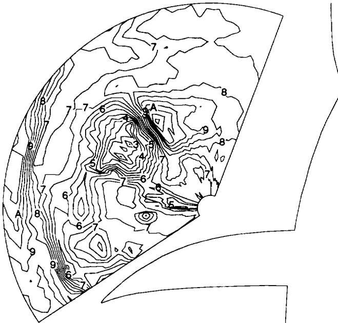
(d) Normalized axial velocity contours.
