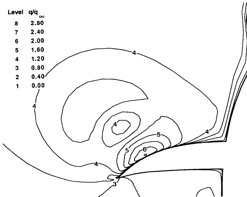
(d) Dynamic pressure contours, computational solution.
