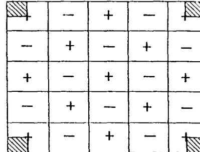
(d) corner mode radiation k < k_m, k < k_n
