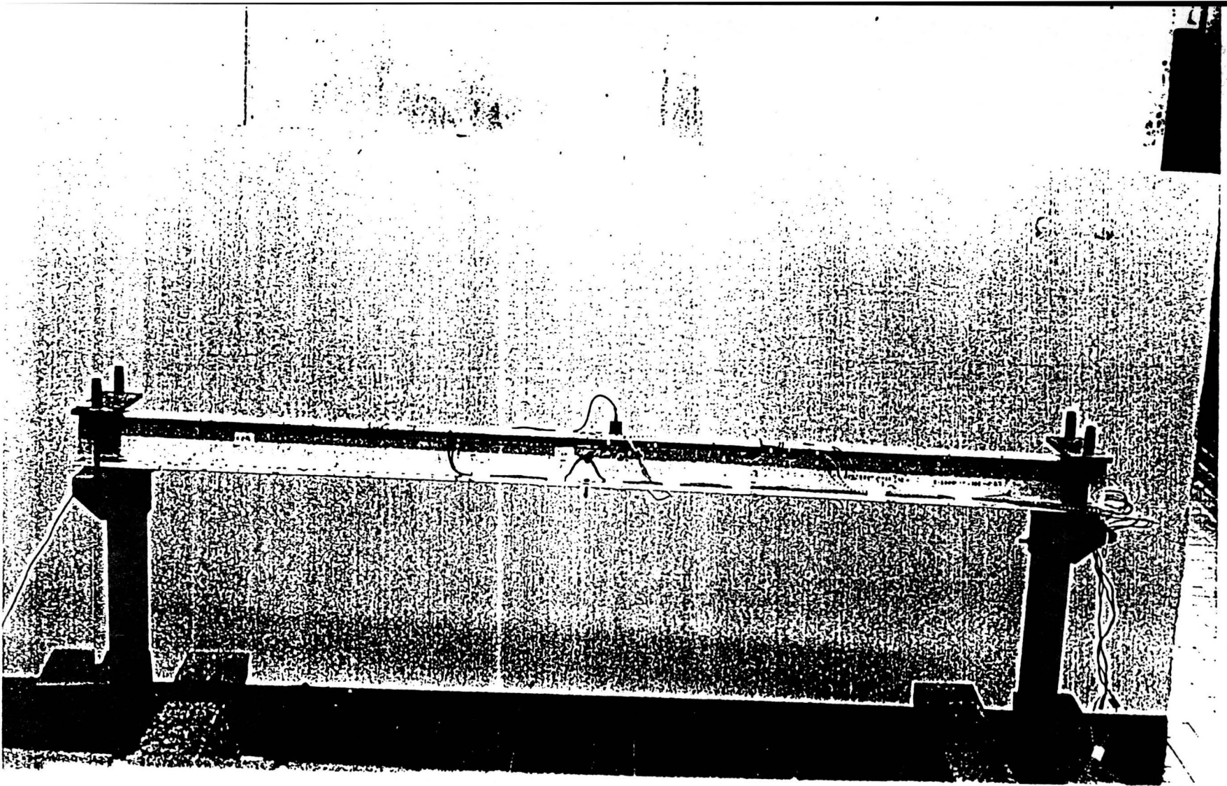
SPECIMEN N. 4 (FRAME)
