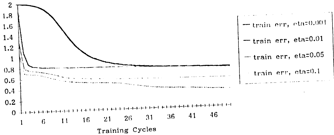
Training Error vs. ETA
