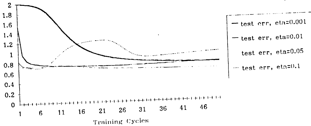
Test Error vs. ETA
