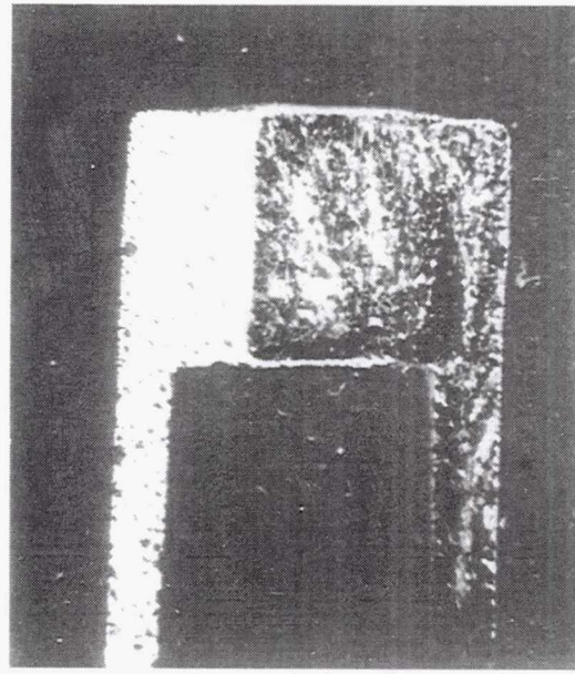
(d) Test time = 56 hours, maximum test temperature = 1322 °C.
