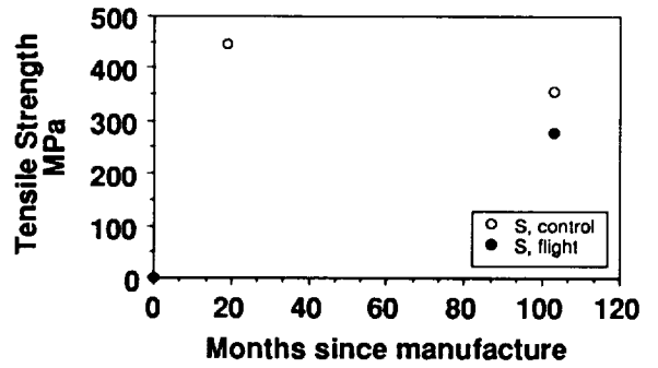
Fig. 20. Group 7: \pm 20^\circ , 0% contact
