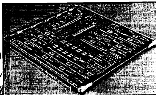
Venus
