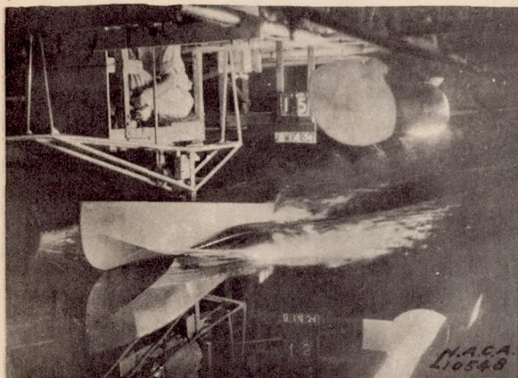
12.0 f.p.s. \tau = 7^\circ \Delta = 100 lb.
