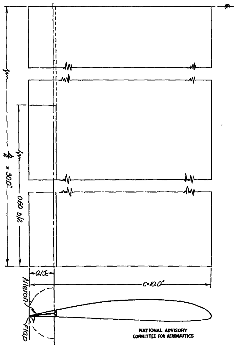
(b) 0.15c flap and aileron.
