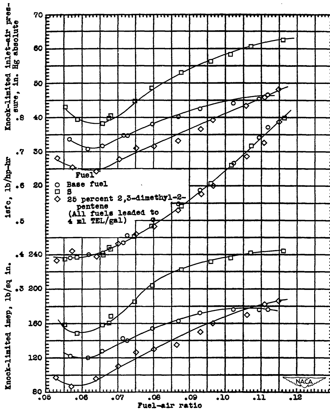
(d) 2,3-Dimethyl-2-pentene.
