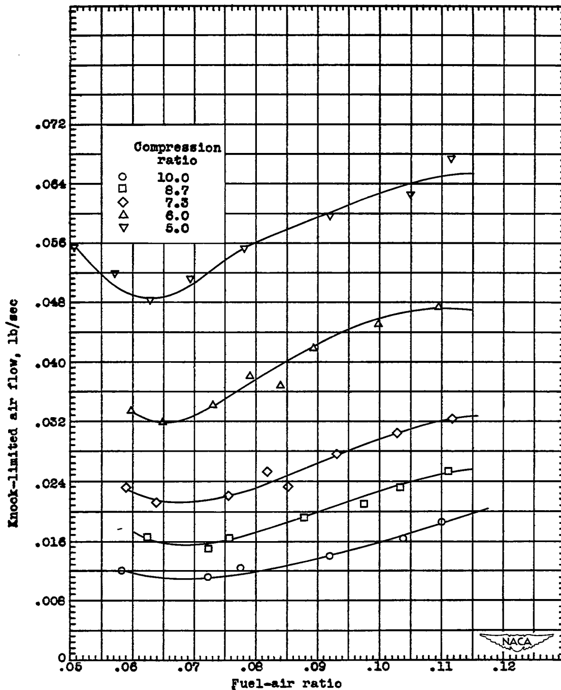
(d) 2,3,4-Trimethyl-2-pentene.
