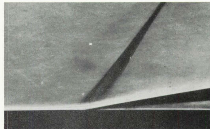
(d) Laminar boundary layer; M_1 = 1.55.
