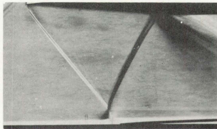
(d) Regular reflection.
