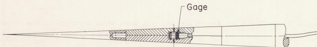
(d) Conical supersonic survey probe.
