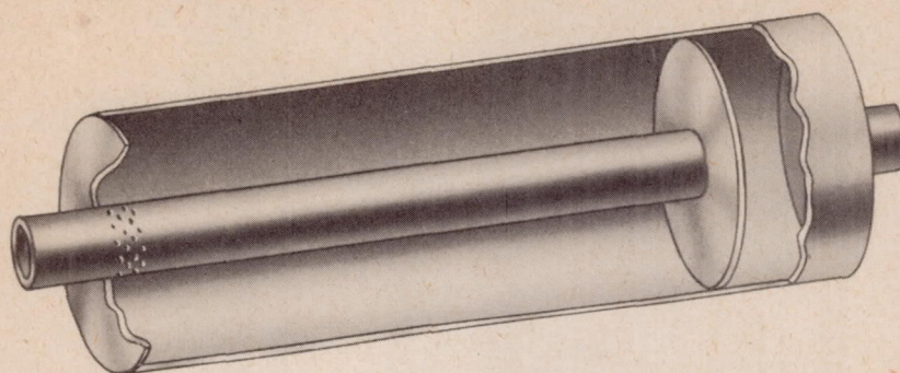
(d) Combination of a resonator and an expansion chamber (muffler 71).
