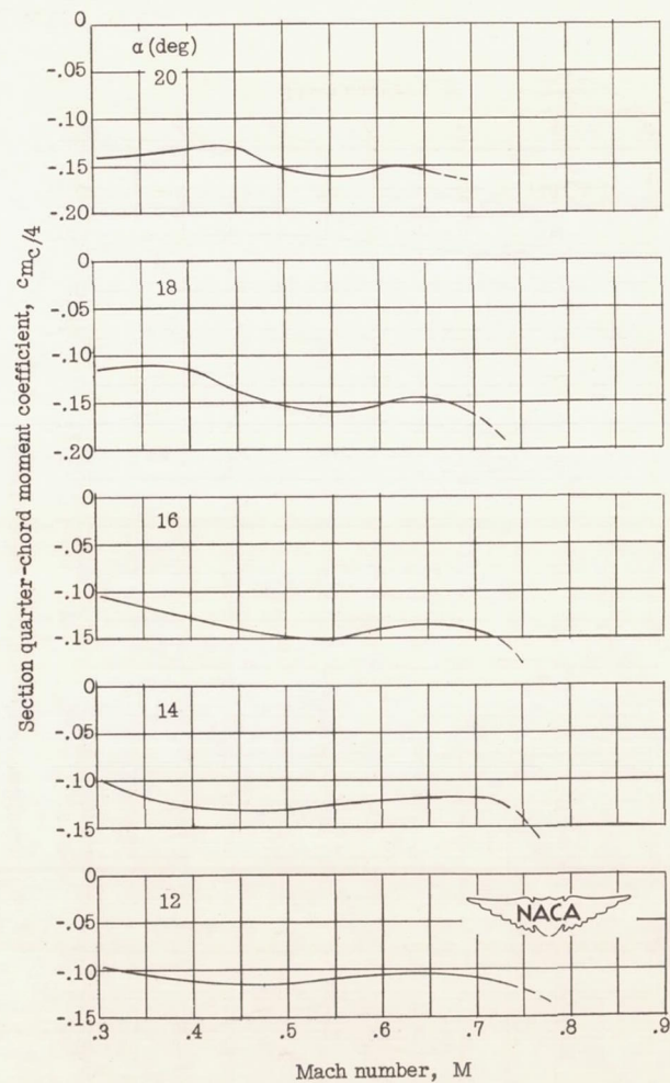
(g) W-3 airfoil.
