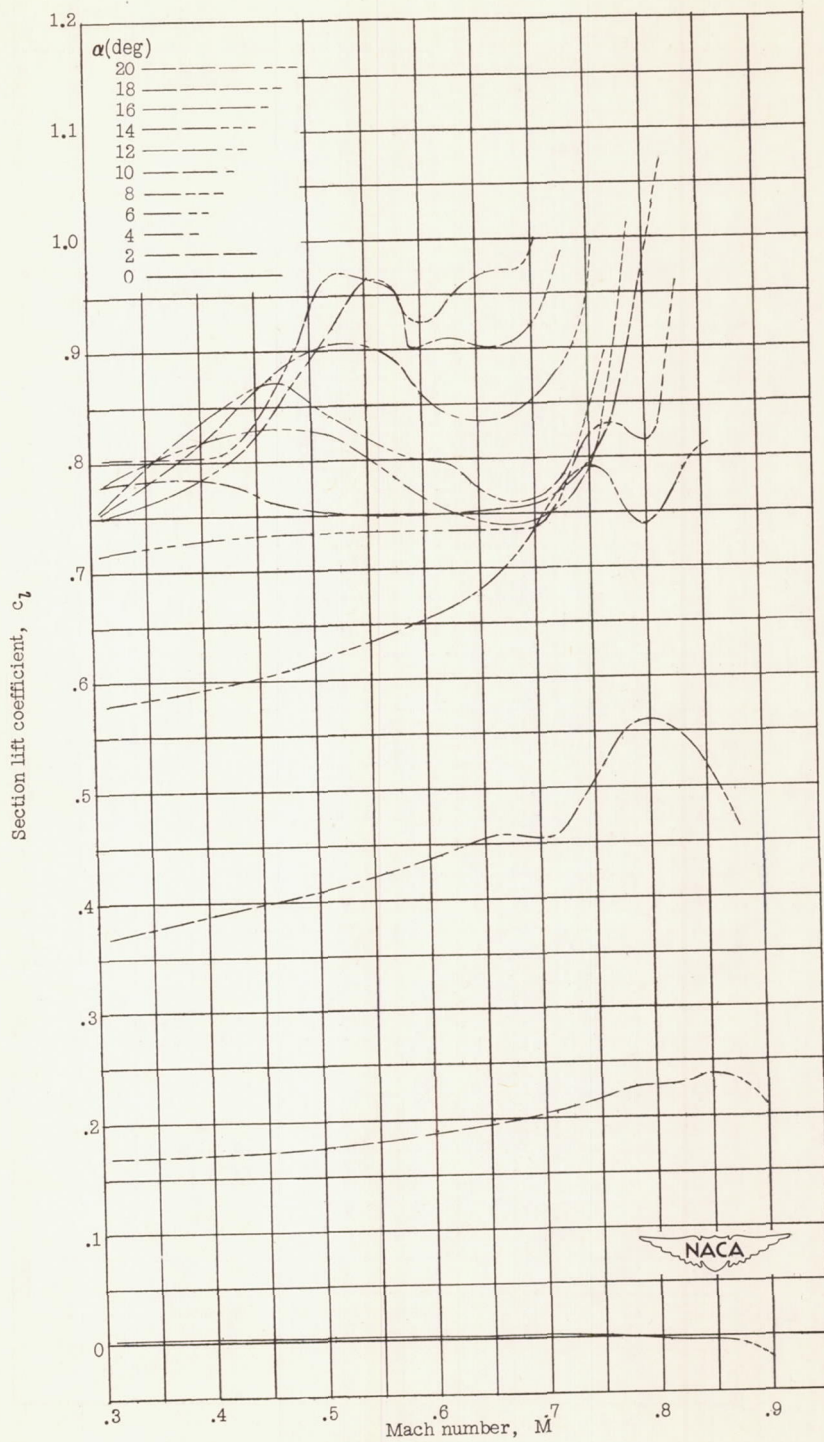
(d) C-3 airfoil.
