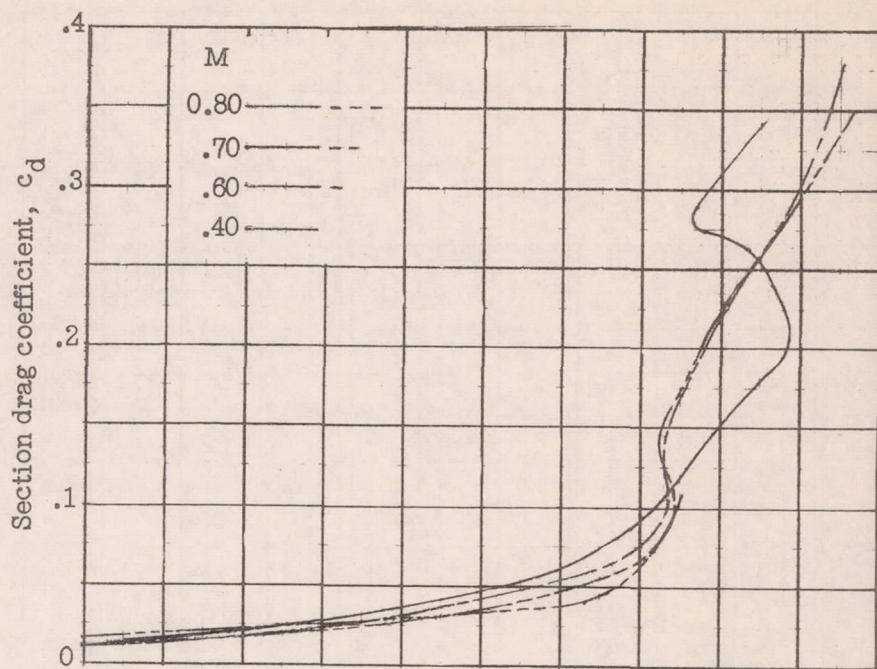
(g) W-3 airfoil.
