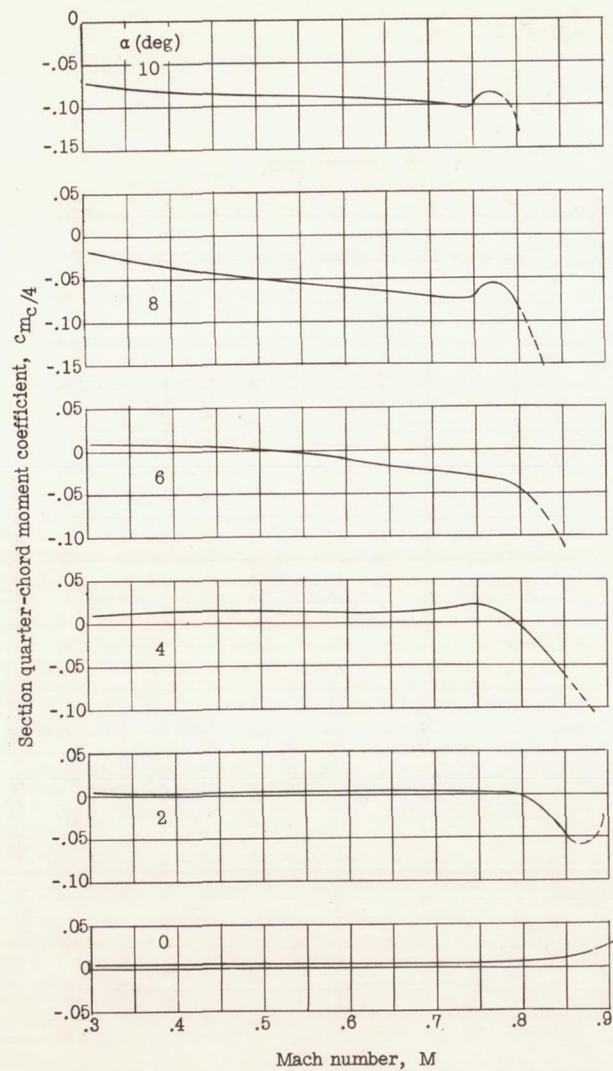
(g) W-3 airfoil.
