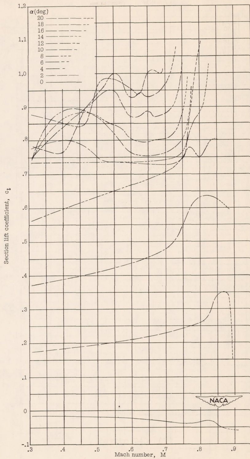
(g) W-3 airfoil.
