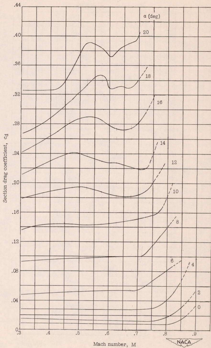
(d) C-3 airfoil.
