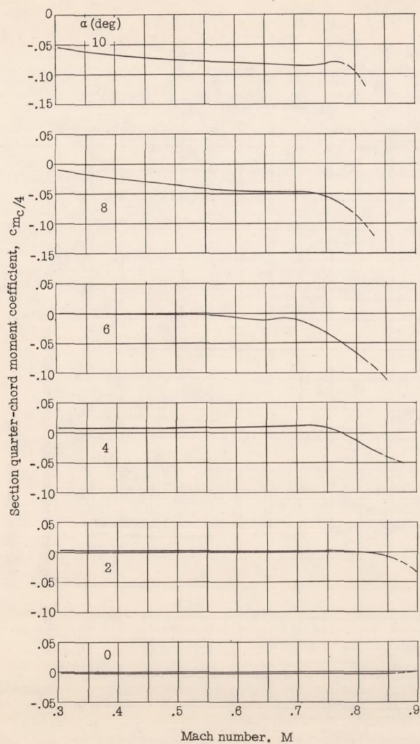
(d) C-3 airfoil.
