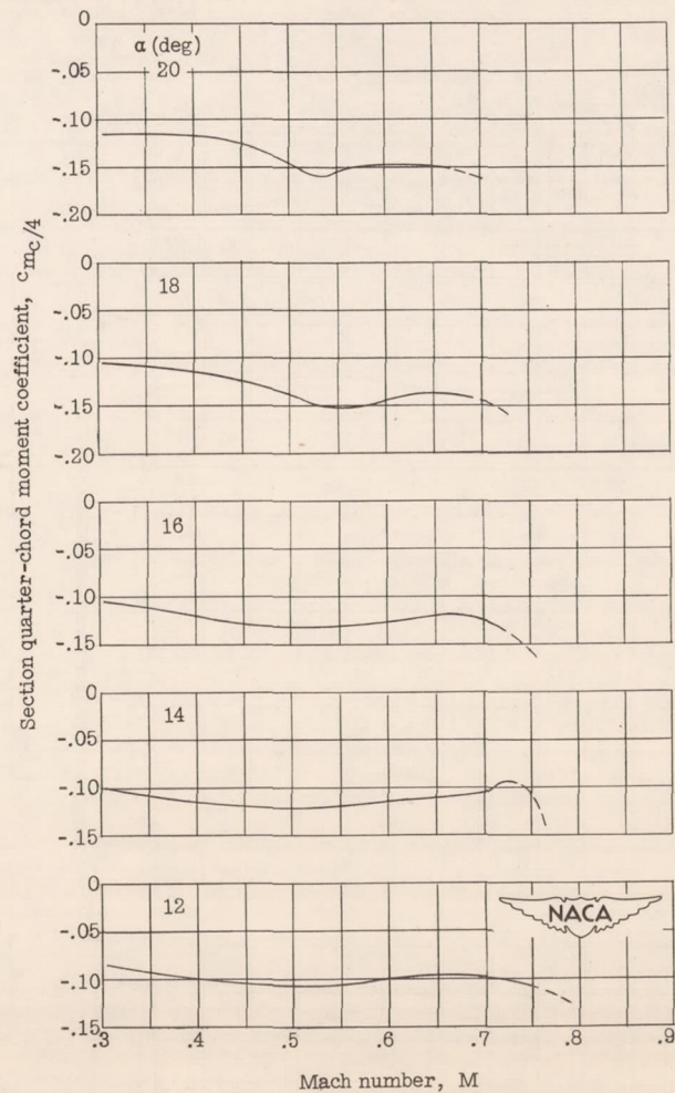
(d) C-3 airfoil.
