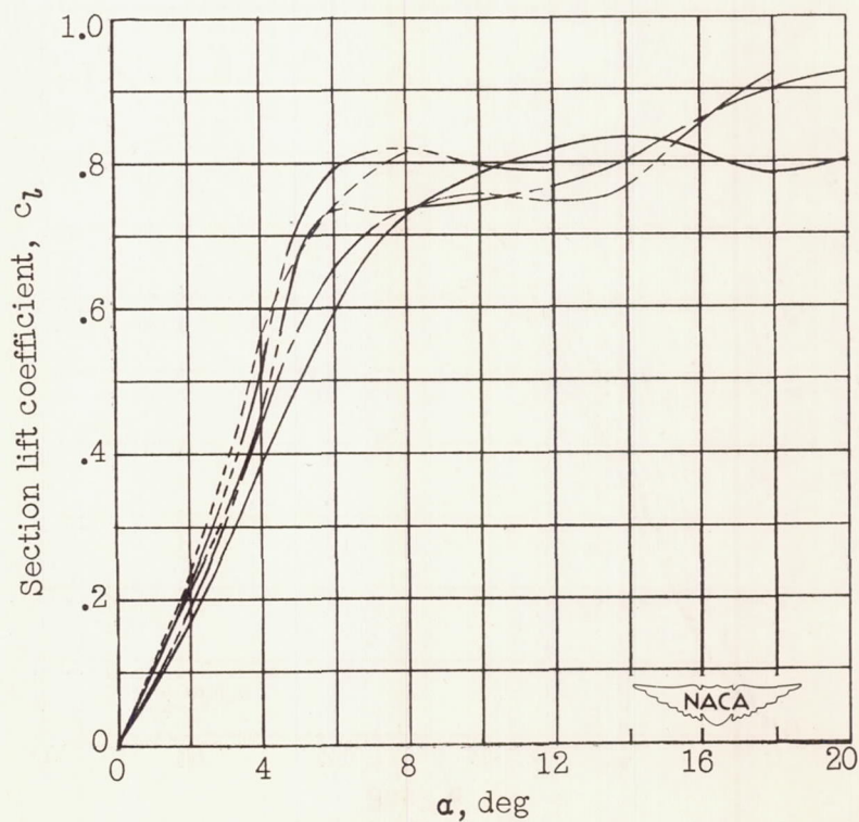
(d) C-3 airfoil.
