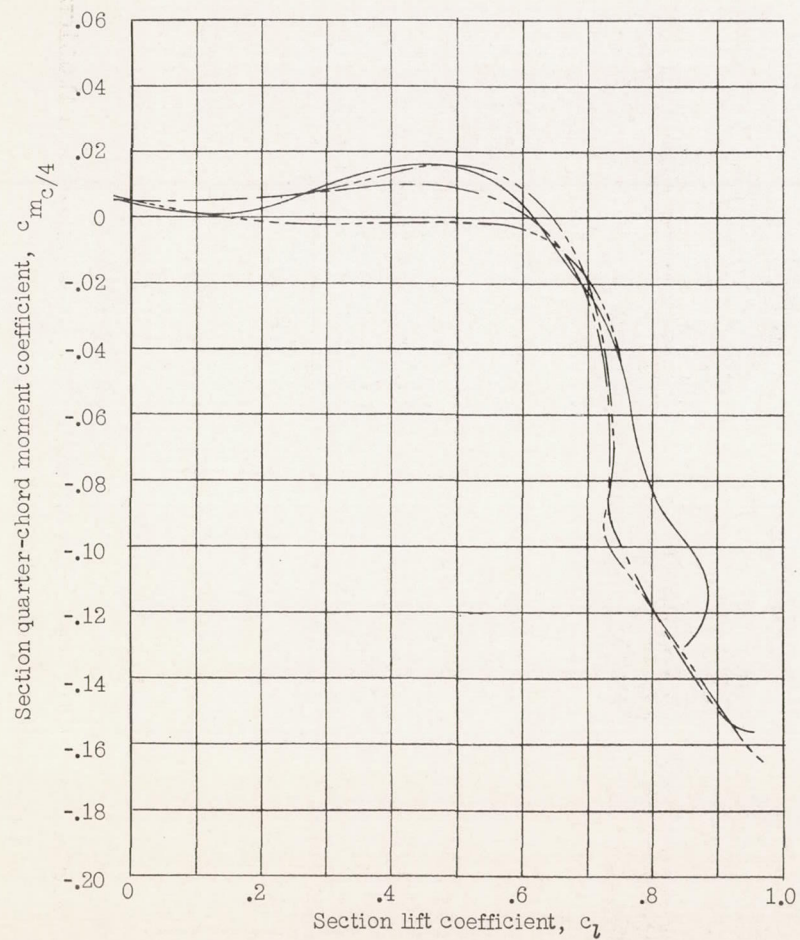
(g) W-3 airfoil.
