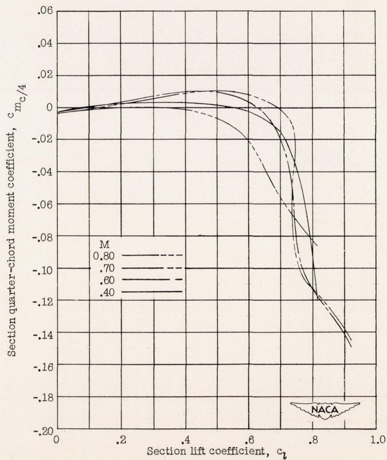
(d) C-3 airfoil.
