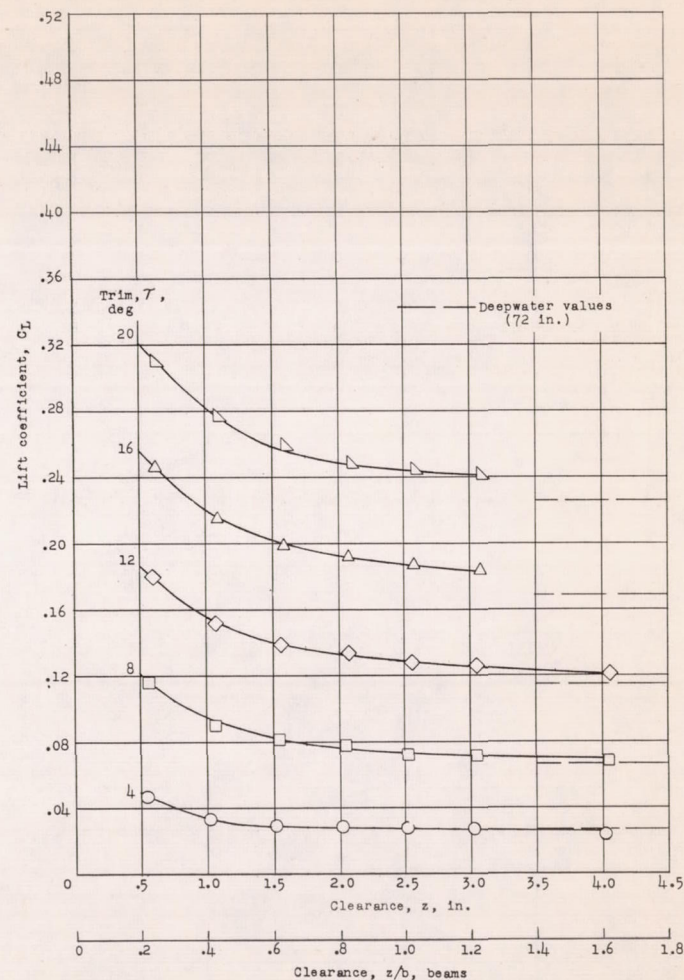
(d) Mean wetted length l_m = 8 inches ( l_m/b = 3.2 ).
