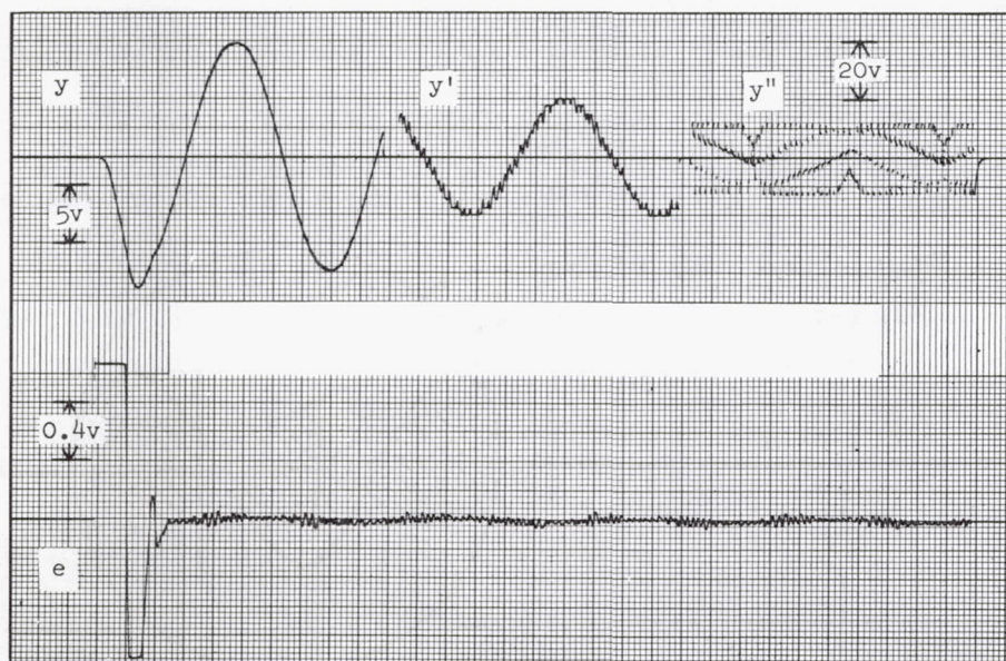
(b) Nonlinear system; 12-volt y'' limit.
