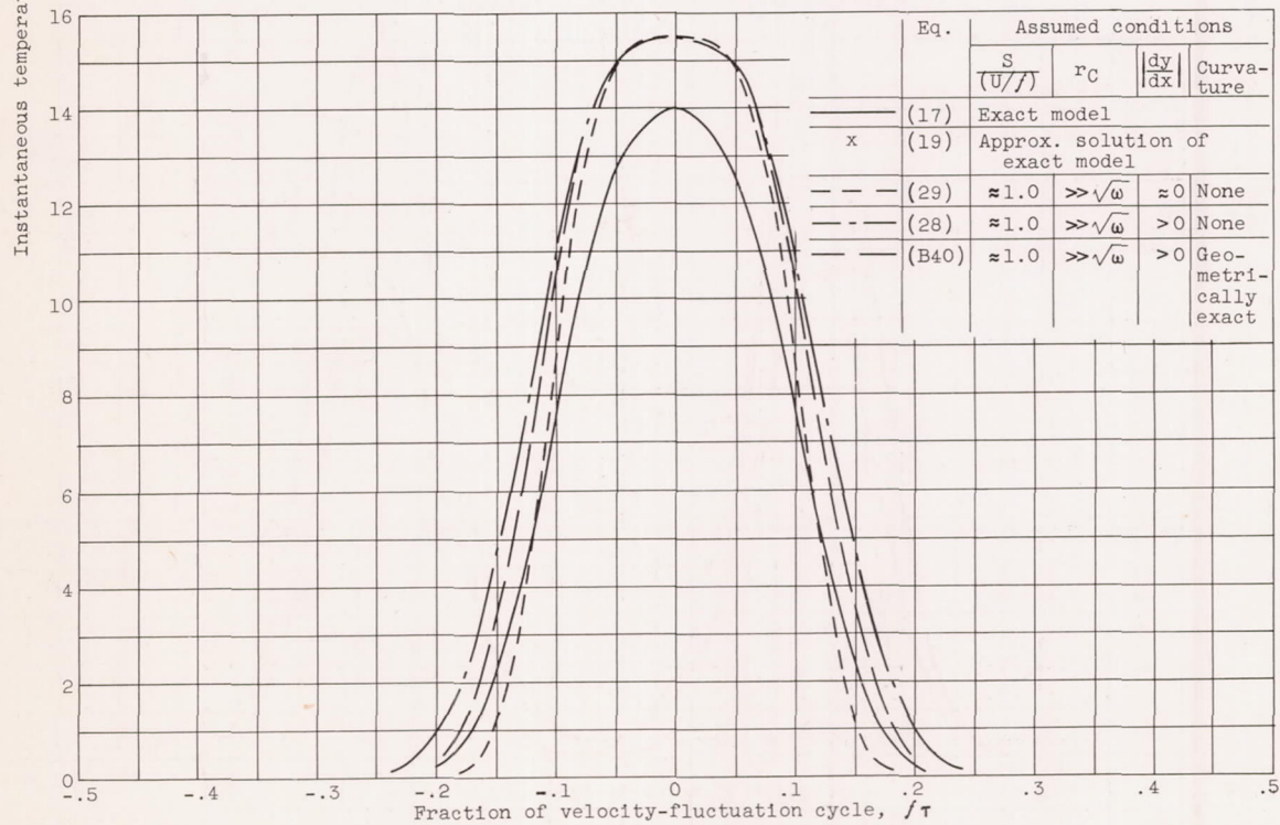
(d) Temperature-time variation at Y/Y_{max} = 1.0 .
