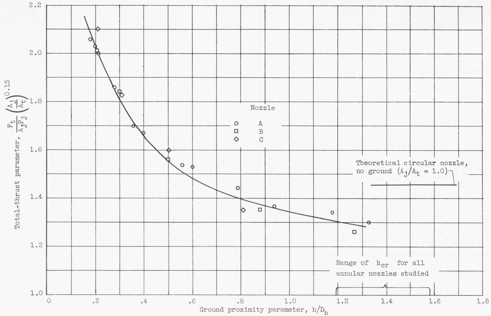
(d) Nominal nozzle pressure ratio, 2.5.
