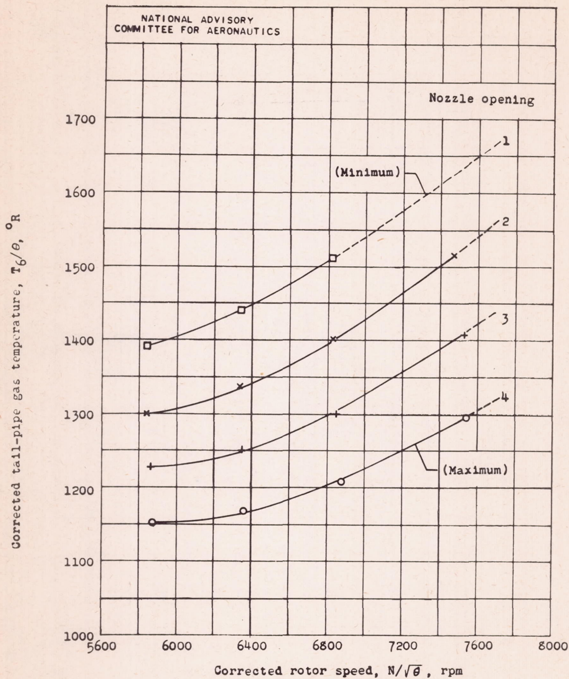
(d) Tail-pipe gas temperature.
